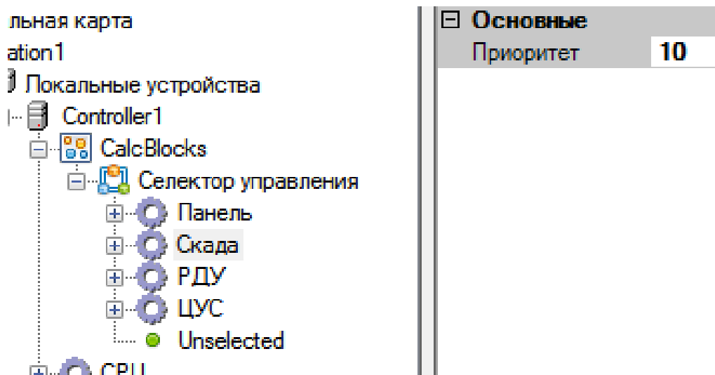
Рисунок 139. Задание приоритета управления
