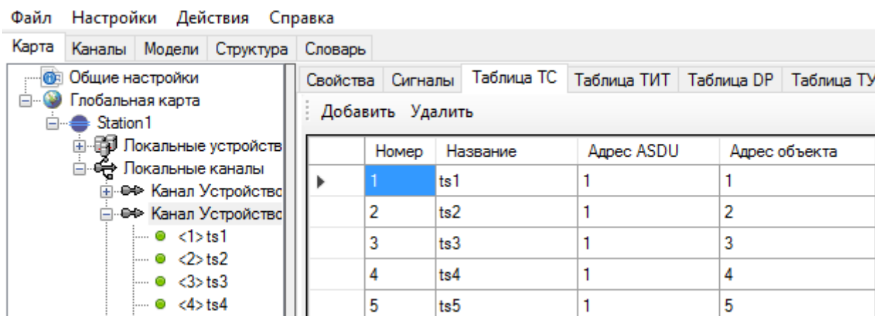
Рисунок 247. Настройки адресации переменных канала связи МЭК60870-5-101
