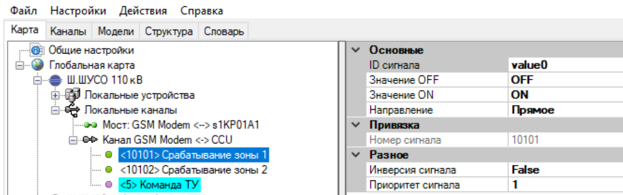
Рисунок 187. Настройка переменных к каналу от устройства «CCU»
