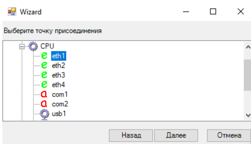
Рисунок 202. Выбор порта на контроллере для связи с IED Modbus TCP
