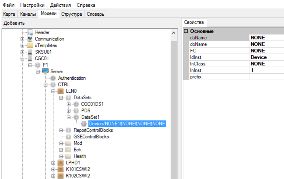
Рисунок 362. Объектная модель. Создание ссылки на объект данных в наборе данных
