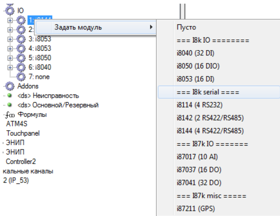
Рисунок 51. Добавление модуля контроллера
