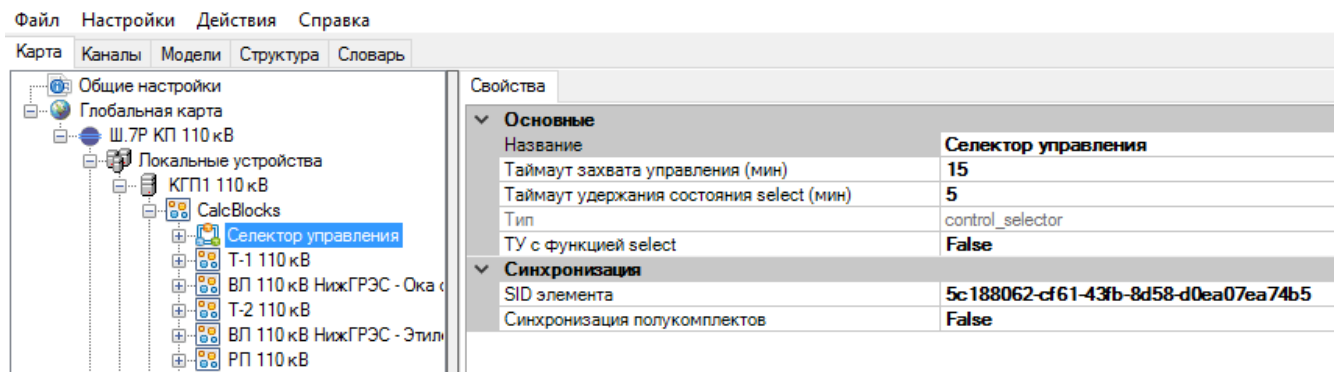
Рисунок 140. Параметры селектора управления
