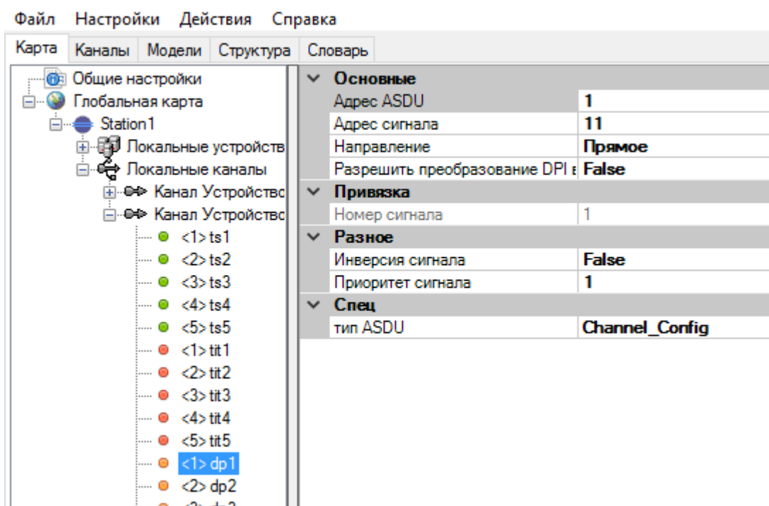
Рисунок 246. Настройки переменных канала связи МЭК60870-5-101
