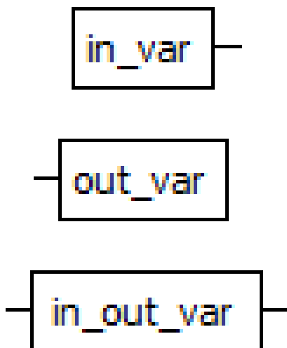
Рисунок 595. Смарт-Дизайнер ПЛК. Программа FBD. Изображение переменной
