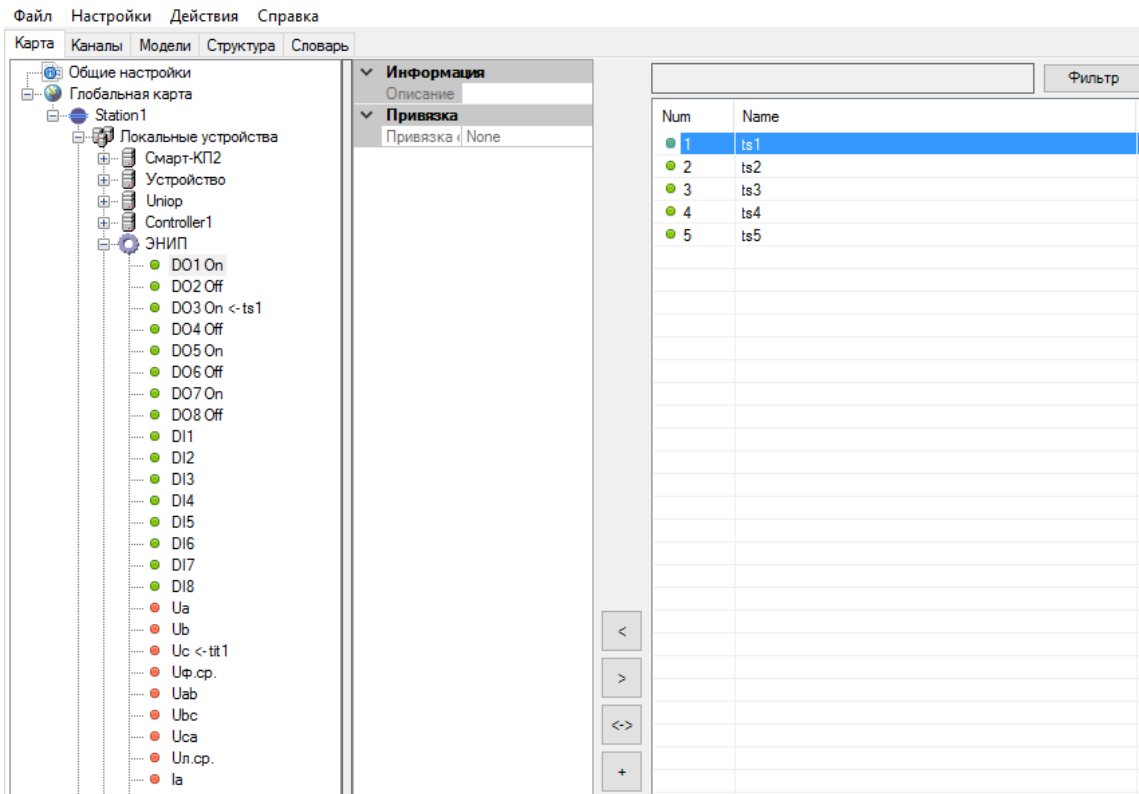
Рисунок 169. Привязка переменных к устройству «ЭНИП»
