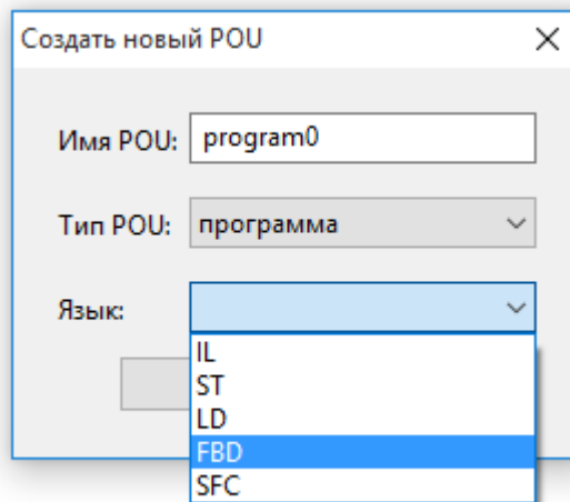
Рисунок 592. Смарт-Дизайнер ПЛК. Выбор языка программы
