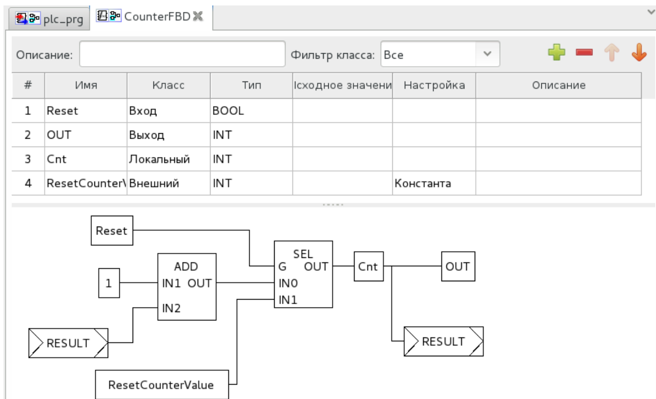
Рисунок 601. Смарт-Дизайнер ПЛК. Программа FBD. Пример использования подключения
