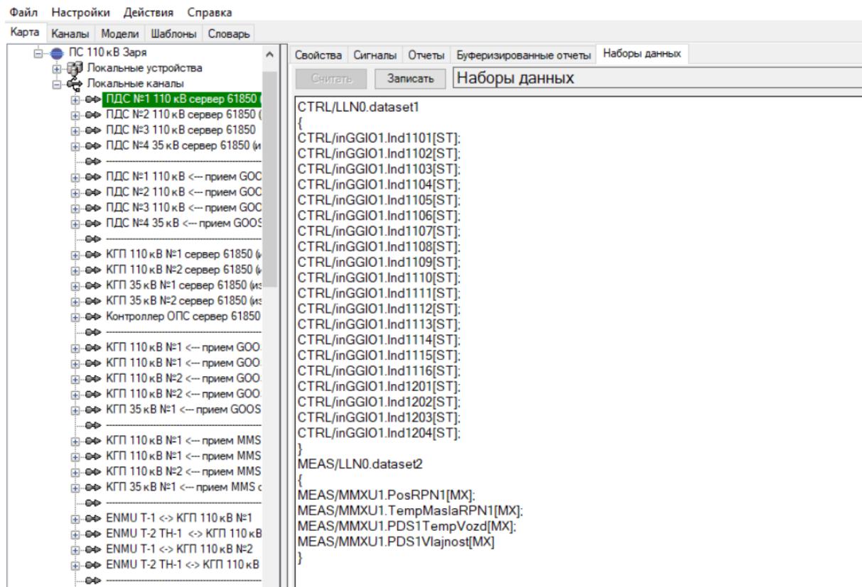
Рисунок 386. MMS сервер Пример записи наборов данных
