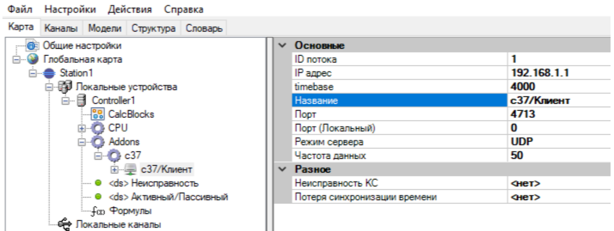
Рисунок 402. С37. Настройка клиента
