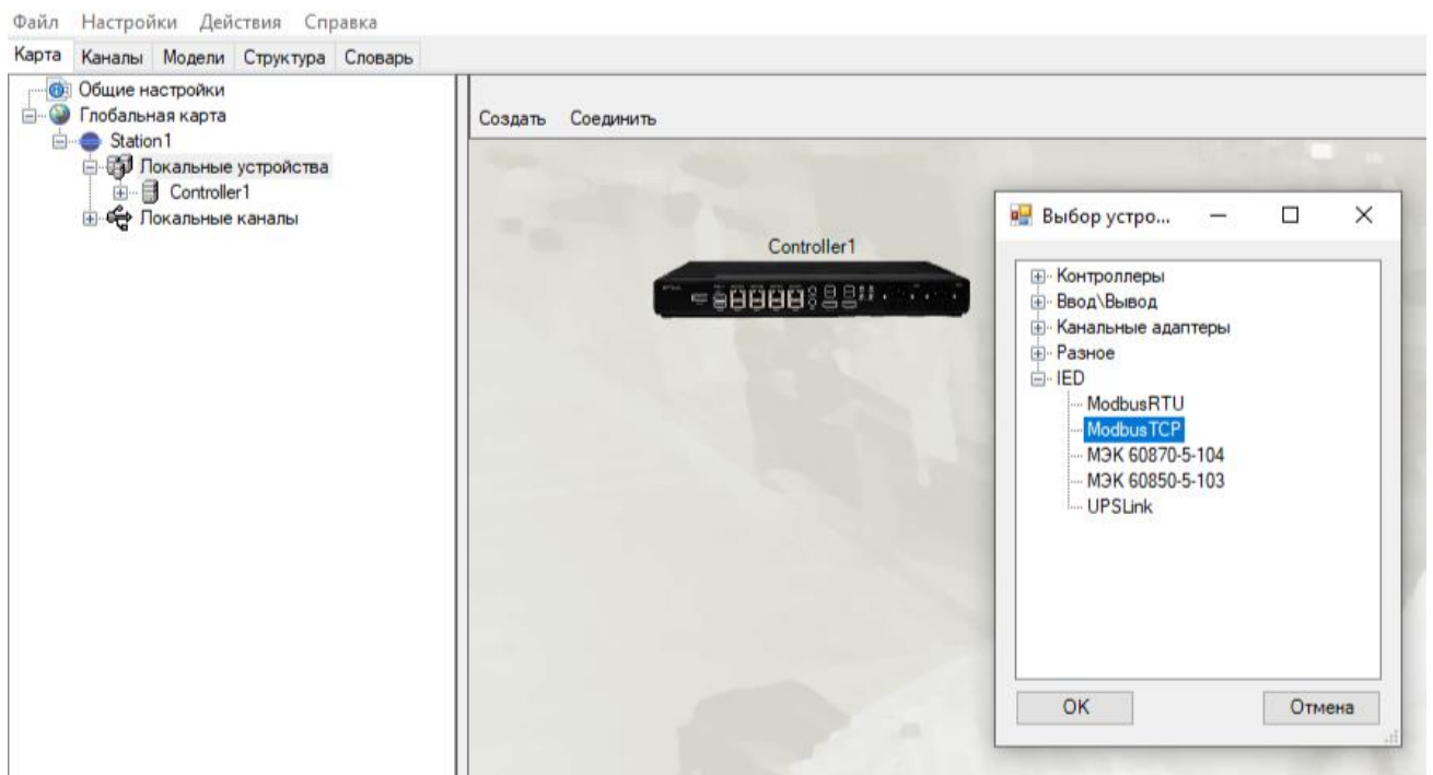
Рисунок 200. Диалоговое окно выбора IED Modbus TCP
