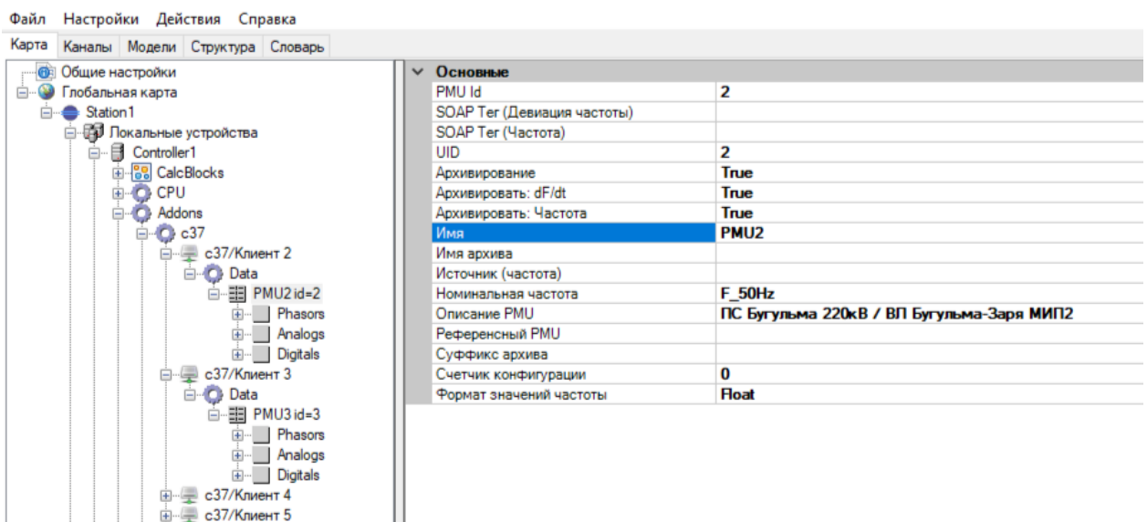
Рисунок 406. С37. Настройка УСВИ
