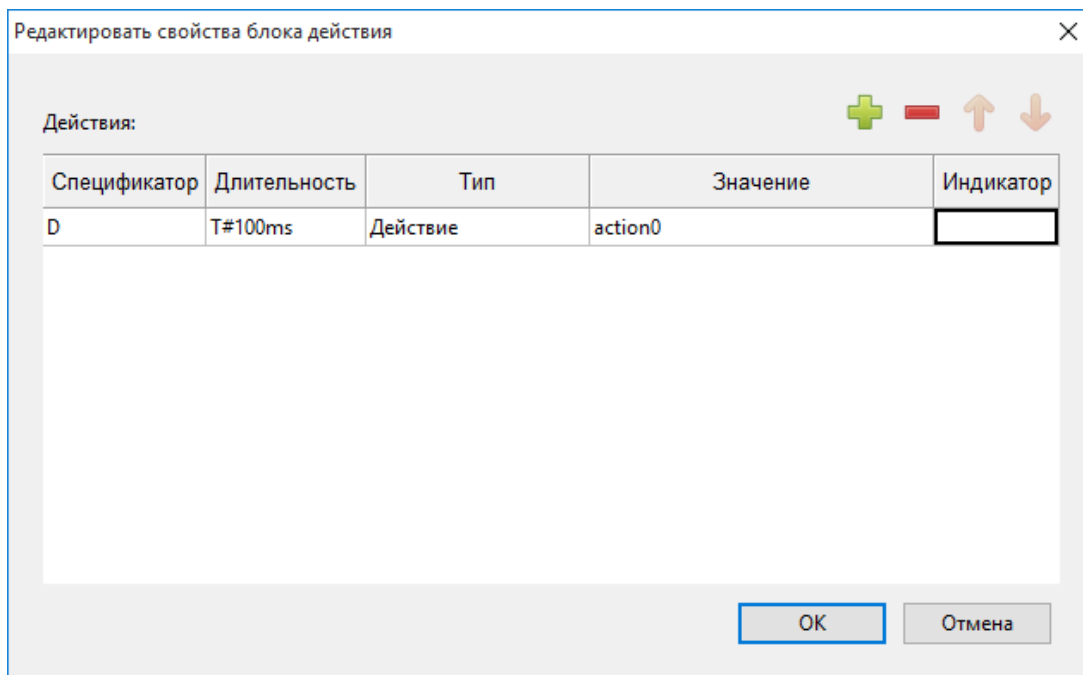
Рисунок 612. Смарт-Дизайнер ПЛК. Программа SFC. Добавление блока действий
