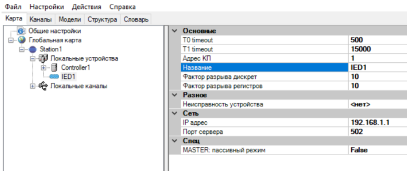
Рисунок 203. Настройка протокола с IED Modbus TCP
