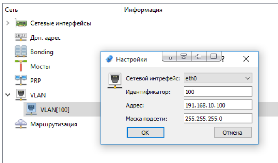
Рисунок 548. Настройка параметров VLAN
