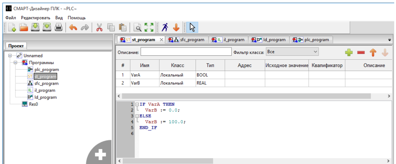
Рисунок 620. Смарт-Дизайнер ПЛК. Программа ST
