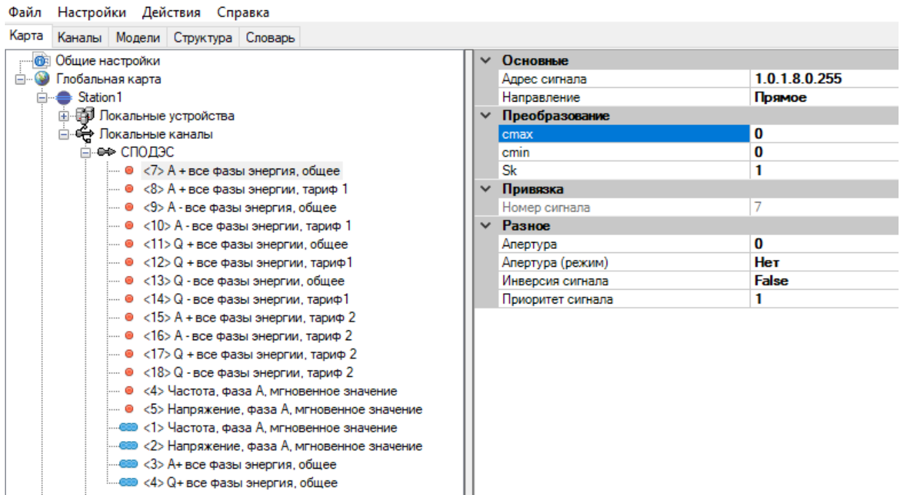
Рисунок 275. Настройки ТИ канала связи DLMS/COSEM
