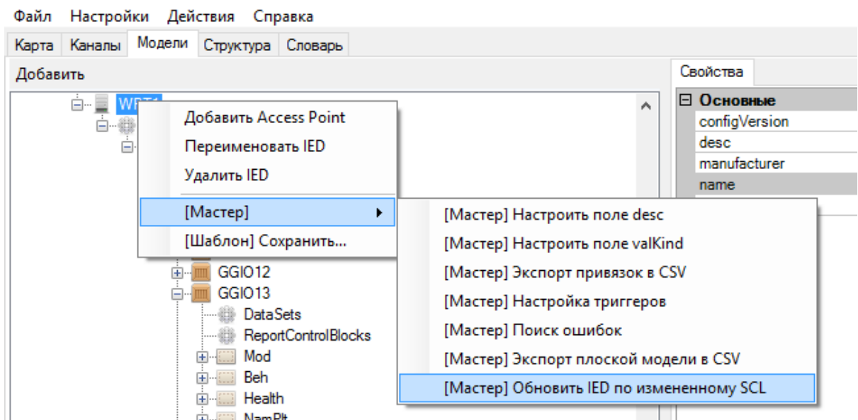
Рисунок 348. Объектная модель. Обновление IED
