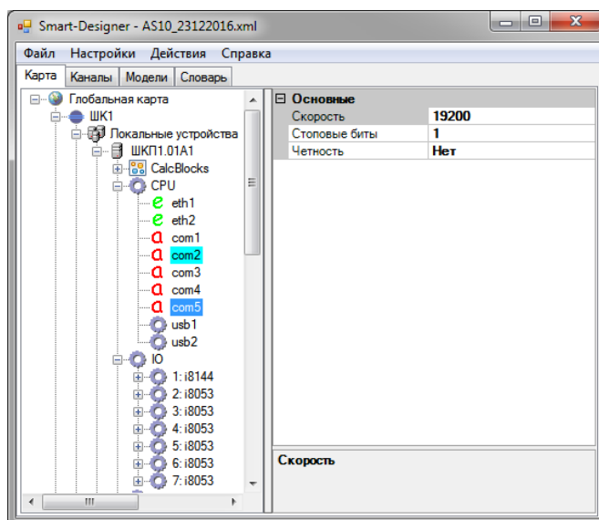
Рисунок 96. Настройка СОМ-порта для панели оператора
