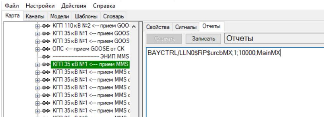
Рисунок 382. MMS клиент. Пример записи наборов данных
