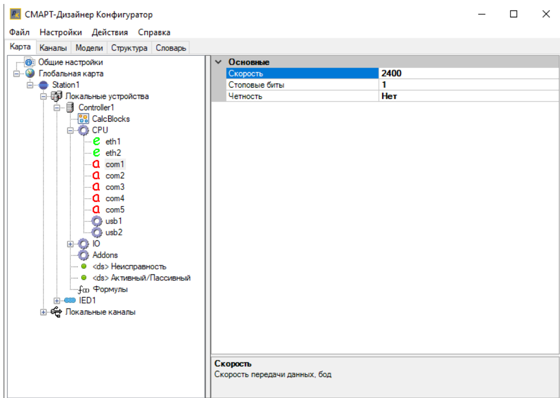
Рисунок 215. Настройка порта на контроллере для связи с IED МЭК 60870-5-103
