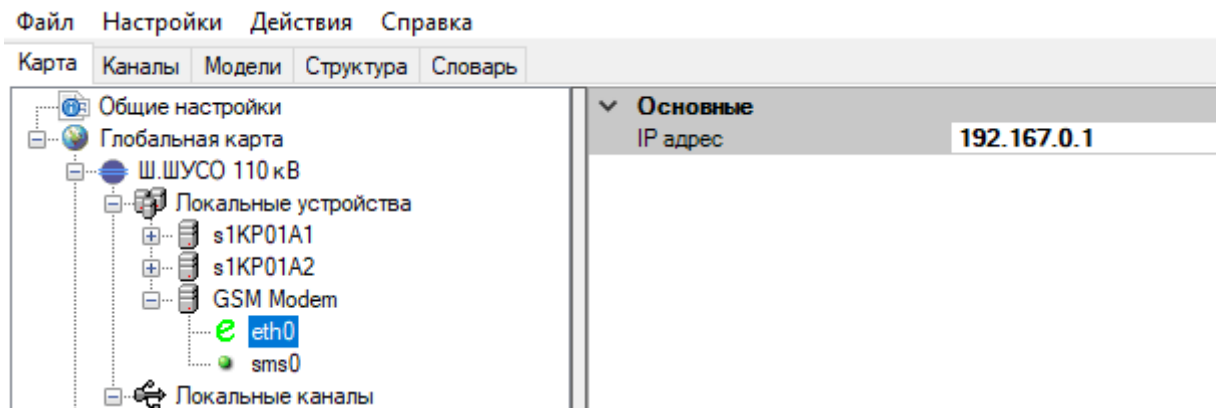
Рисунок 93. Настройка IP-адреса GSM модема
