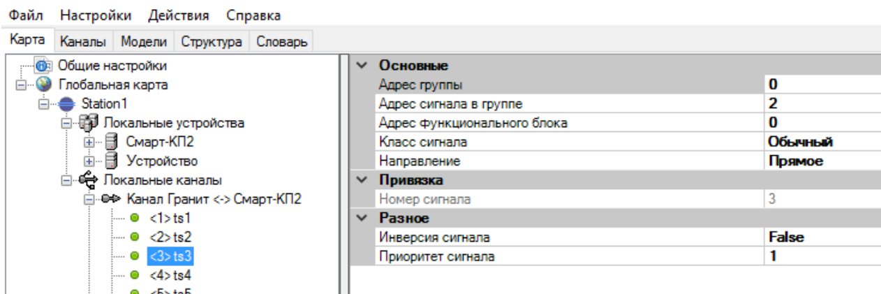
Рисунок 295. Настройки ТС канала связи Гранит
