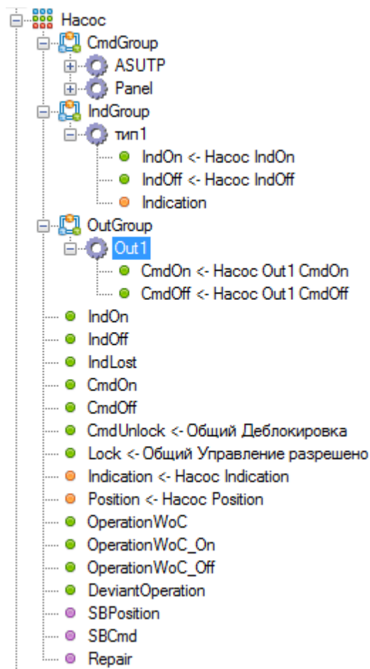
Рисунок 132. Пример создания «Насос»
