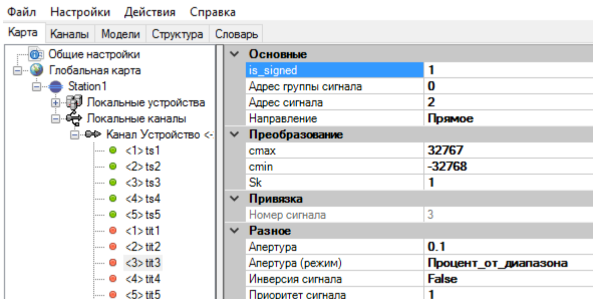
Рисунок 283. Настройки ТИ канала связи Телеканал М2
