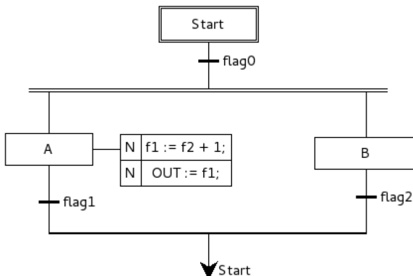
Рисунок 617. Смарт-Дизайнер ПЛК. Программа SFC. Параллельное ветвление
