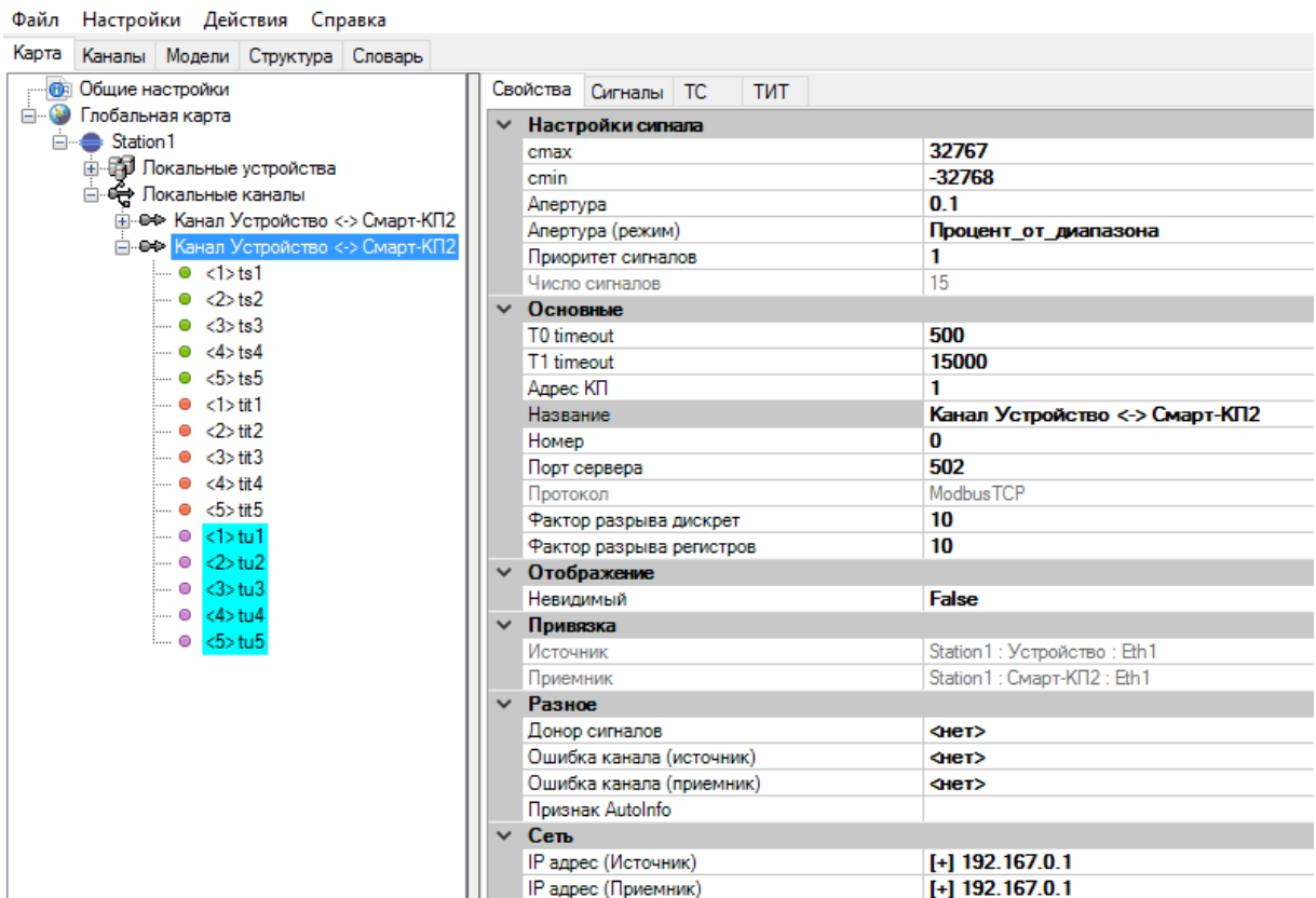
Рисунок 257. Настройки канала связи Modbus TCP
