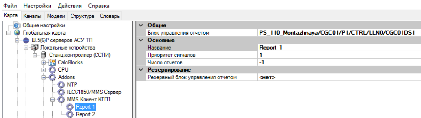
Рисунок 332. MMS клиент. Настройка параметров отчета
