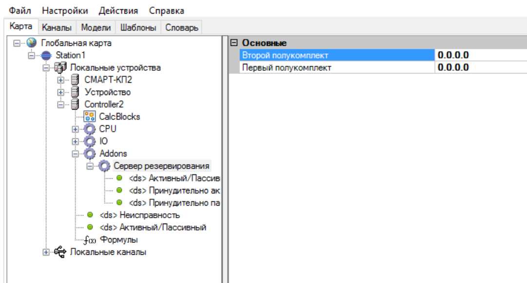
Рисунок 100. Настройки сервера резервирования
