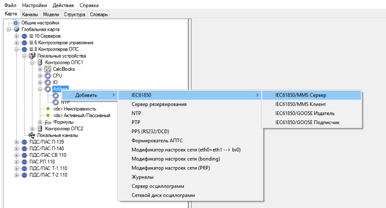
Рисунок 334. Добавление MMS сервера
