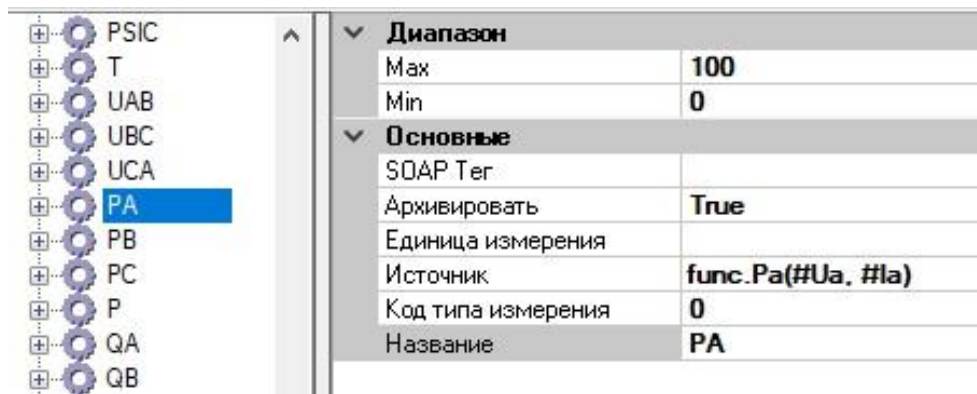
Рисунок 400. С37. Пример уточнения имен
