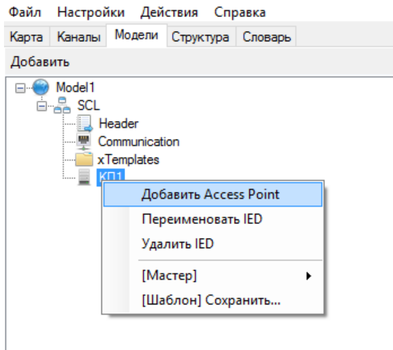
Рисунок 351. Объектная модель. Добавление точки доступа IED-устройства
