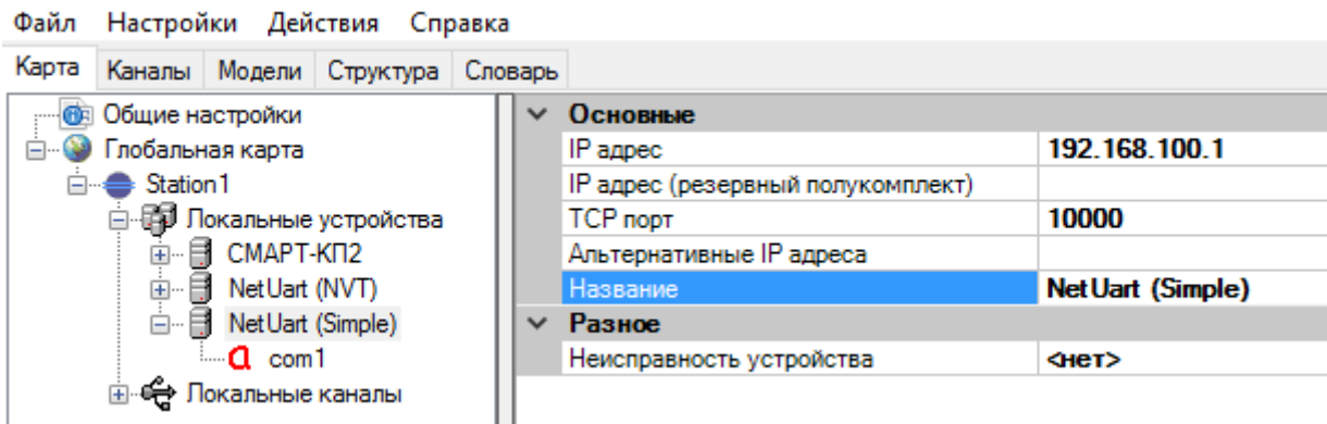
Рисунок 85. Конфигурирование канального адаптера «NetUart»
