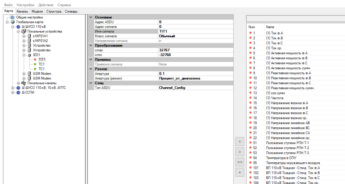
Рисунок 192. Настройка переменных IED устройства
