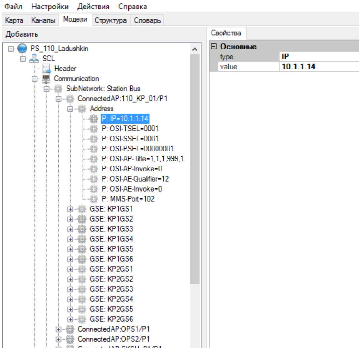
Рисунок 308. Объектная модель. Адрес точки доступа к соединению
