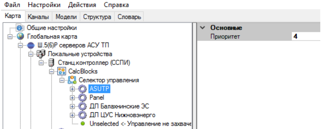
Рисунок 142. Приоритеты групп селектора управления
