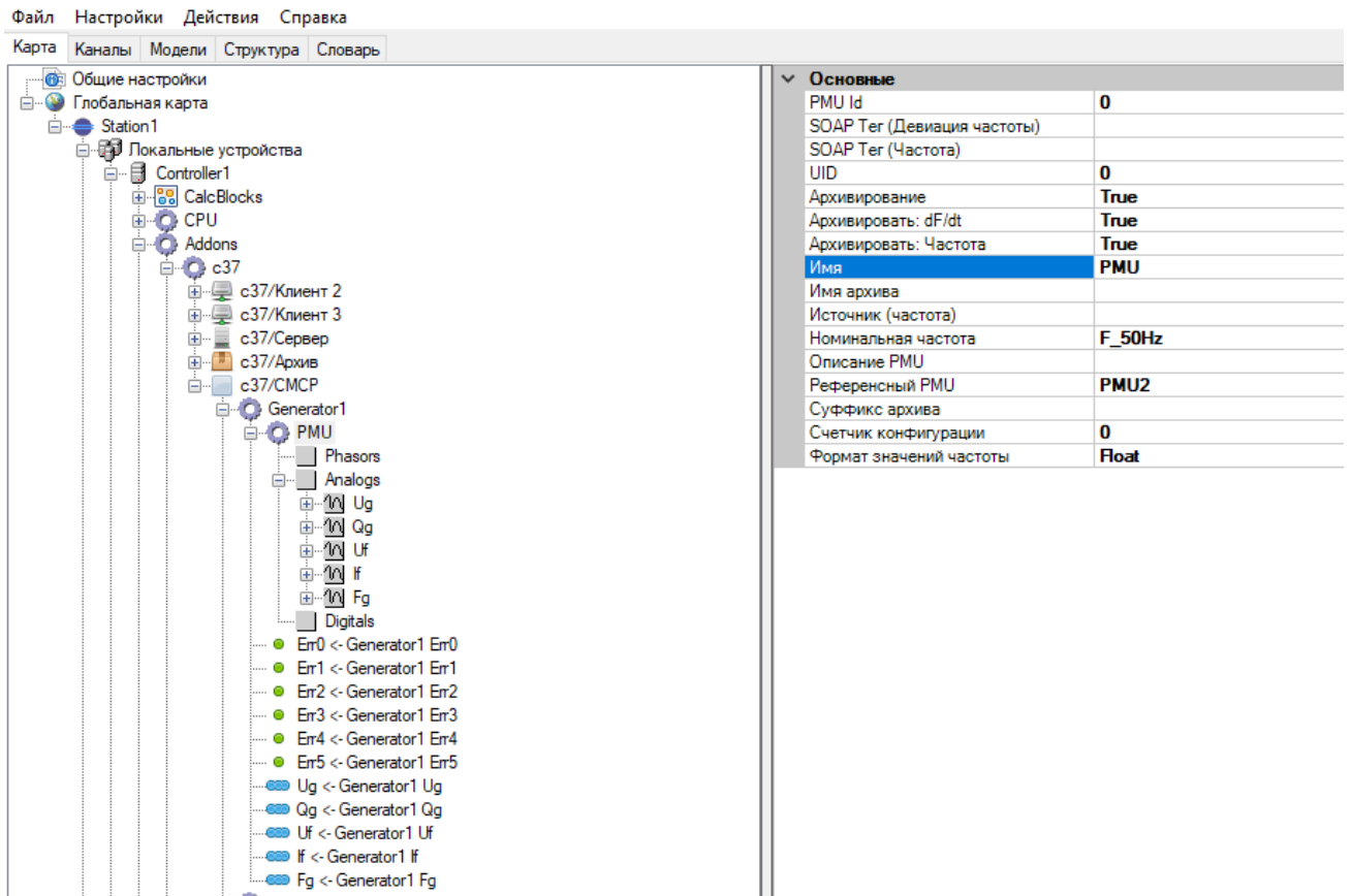
Рисунок 446. С37. Настройка источника УСВИ генератора СМСР
