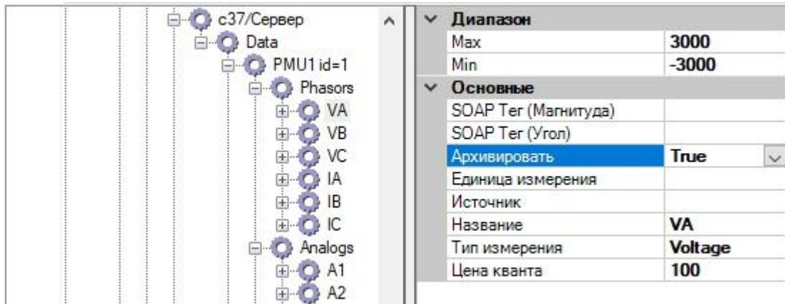
Рисунок 439. С37. Включение параметра VA в архив
