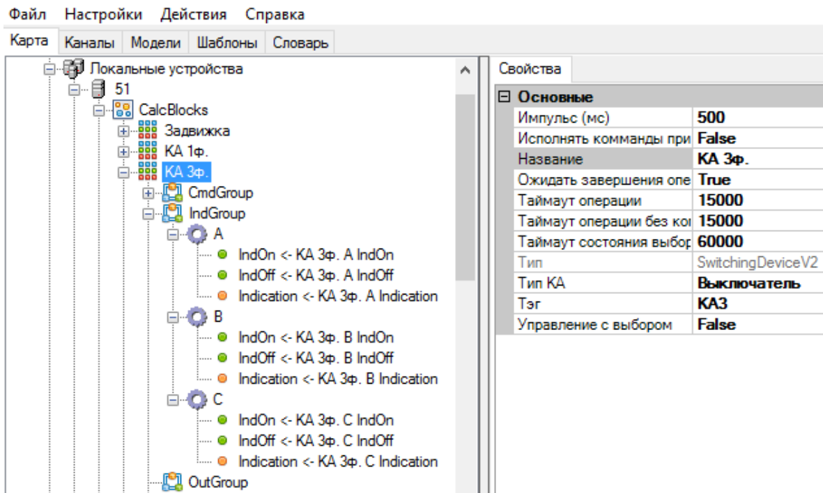
Рисунок 128. Пример трехфазного коммутационного аппарата
