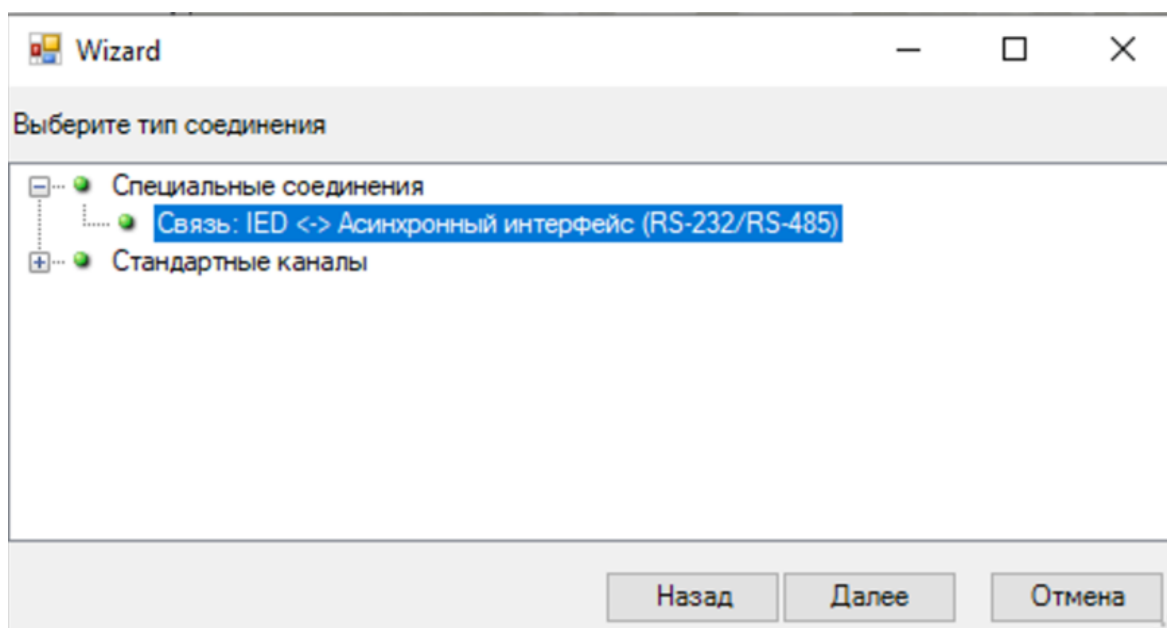
Рисунок 213. Добавление связи с IED МЭК 60870-5-103
