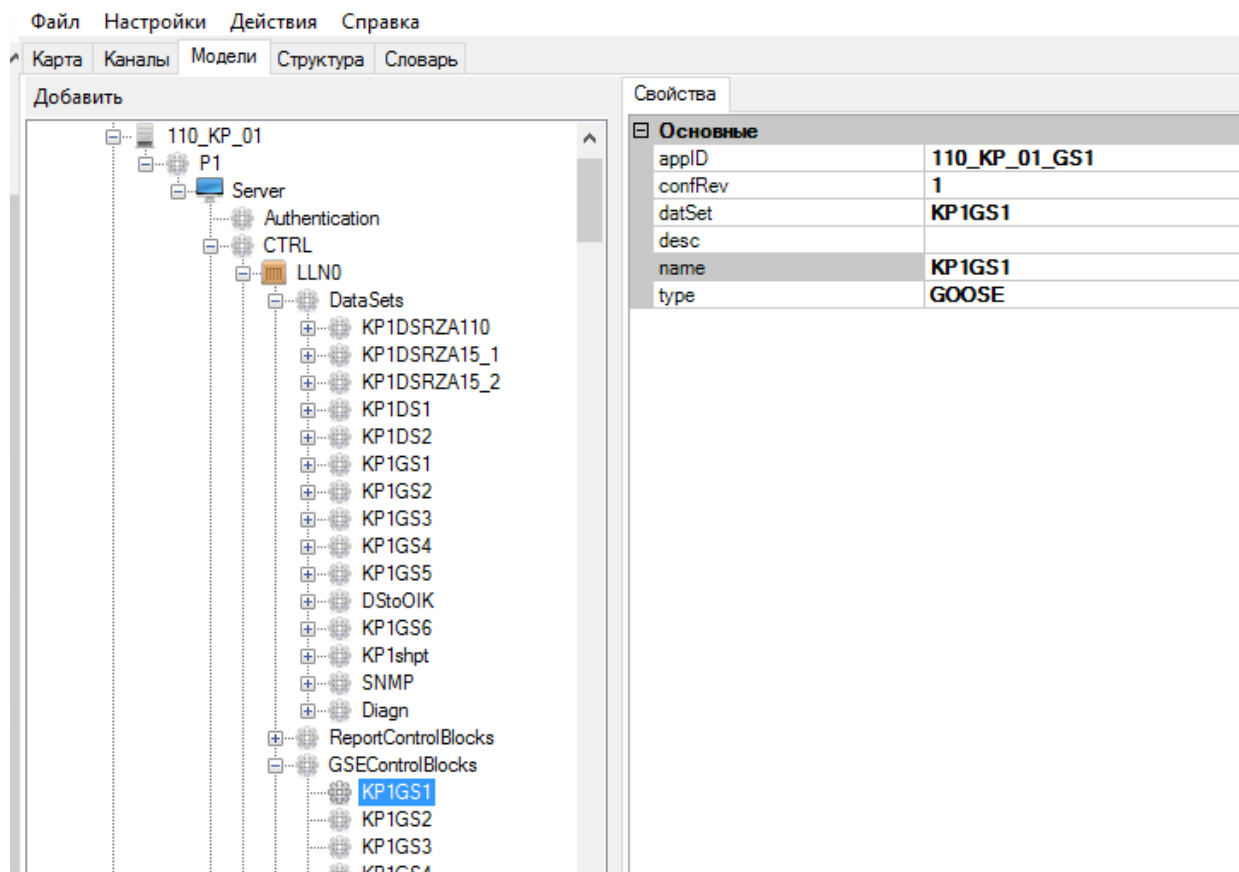
Рисунок 328. Объектная модель. Блок управления GOOSE сообщениями
