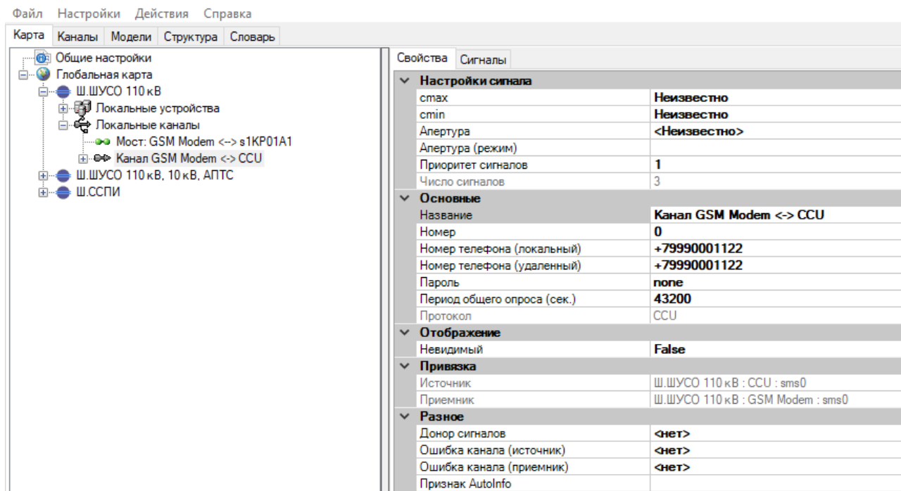
Рисунок 186. Конфигурирование канала связи с «CCU»
