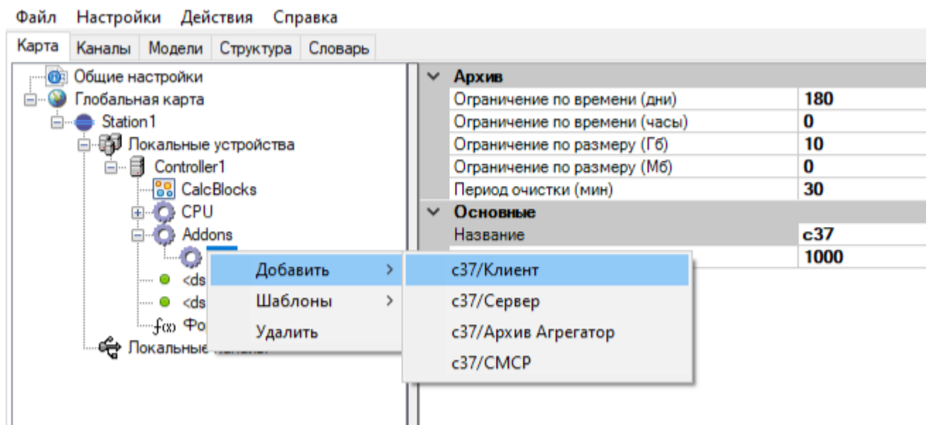
Рисунок 401. С37. Добавление клиента
