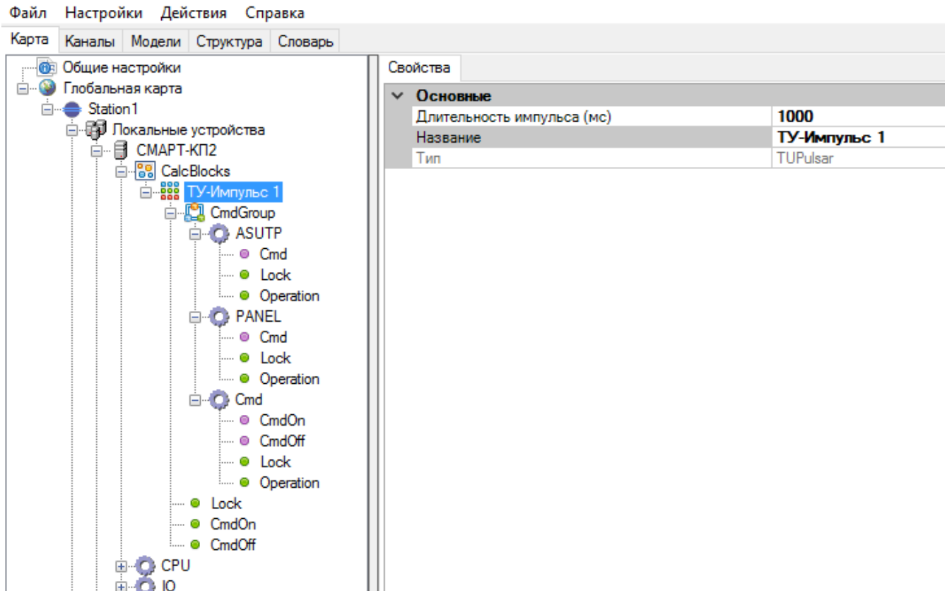
Рисунок 153. Функциональный блок ТУ-импульс
