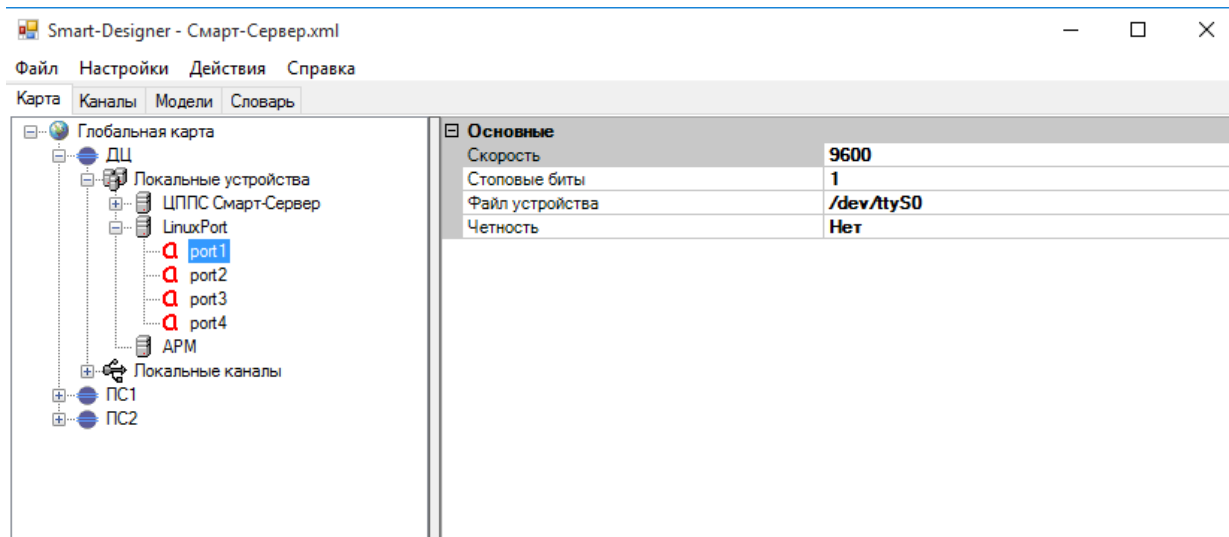
Рисунок 81. Конфигурирование портов канального адаптера «LinuxPort»
