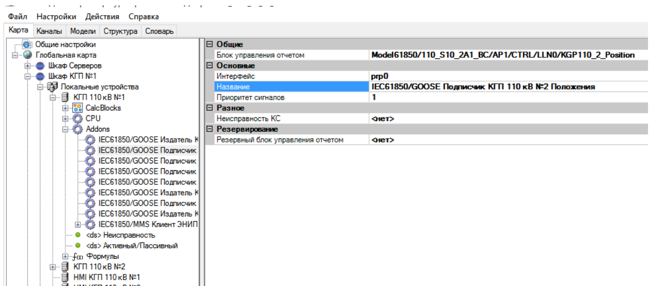
Рисунок 338. Настройка GOOSE подписчика
