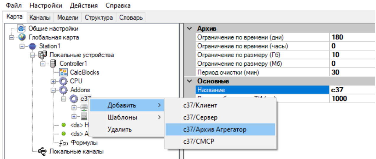
Рисунок 441. С37. Добавление компонента Архив Агрегатор
