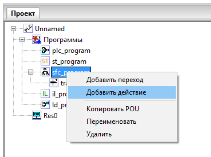
Рисунок 613. Смарт-Дизайнер ПЛК. Программа SFC. Добавление предопределенного действия в дереве проекта
