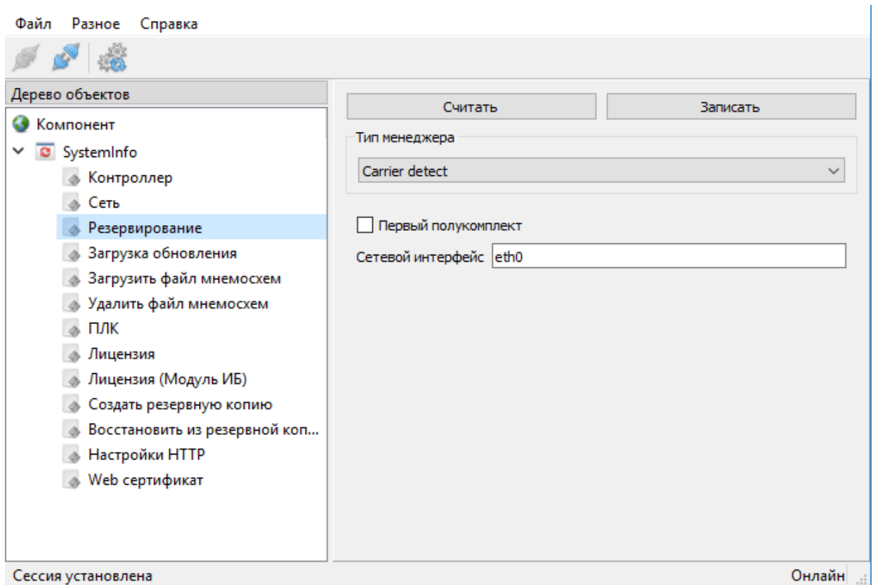
Рисунок 534. Настройки режима «Carrier detect»
