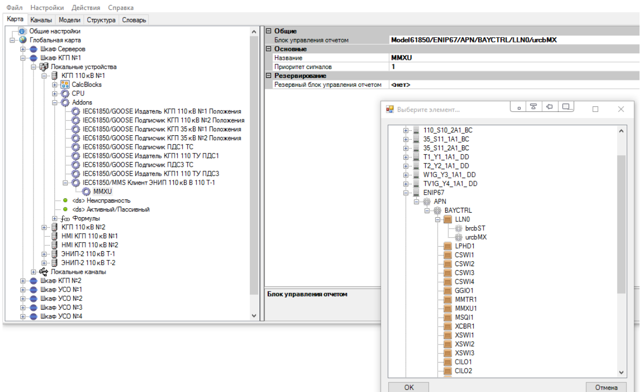
Рисунок 333. MMS клиент. Создание ссылки на отчет
