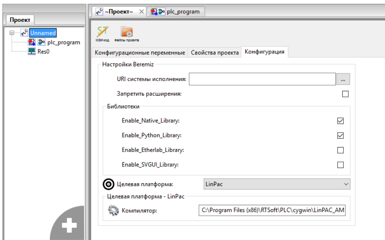
Рисунок 589. Смарт-Дизайнер ПЛК. Выбор целевой платформы
