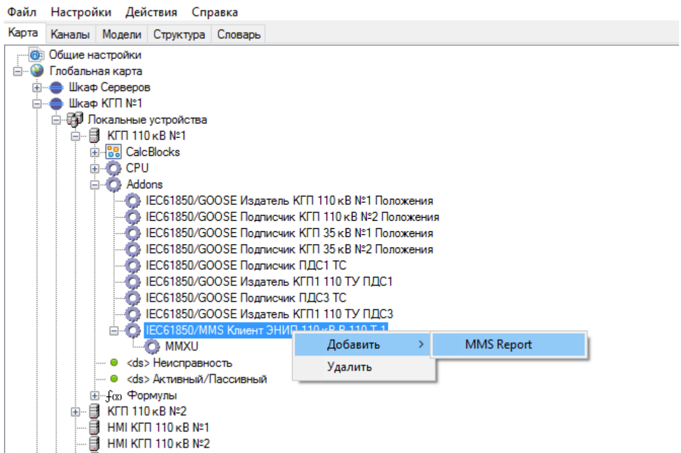
Рисунок 331. MMS клиент. Добавление подписки на отчет
