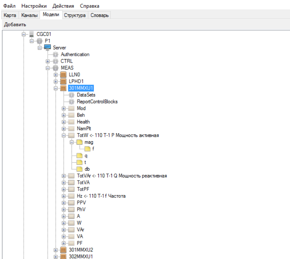
Рисунок 357. Объектная модель. Добавление логического узла MMXU
