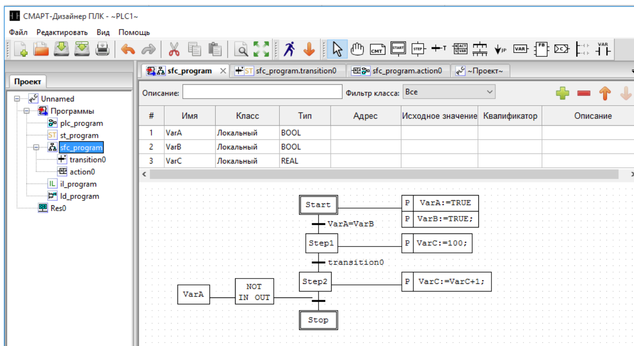
Рисунок 607. Смарт-Дизайнер ПЛК. Программа SFC
