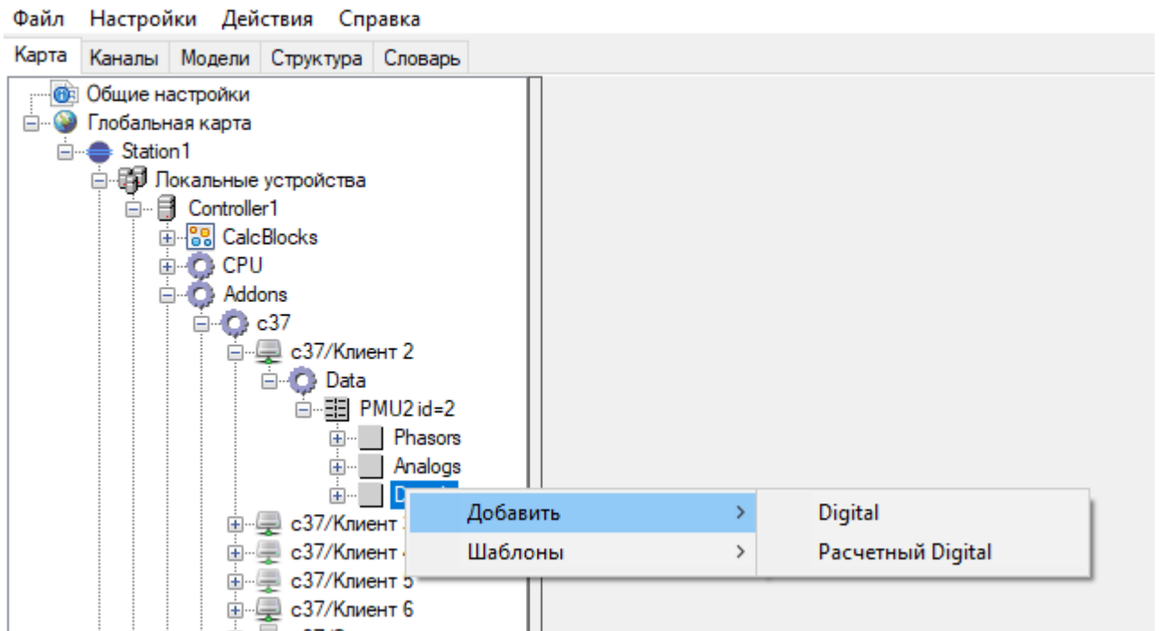
Рисунок 413. Добавление дискретной величины
