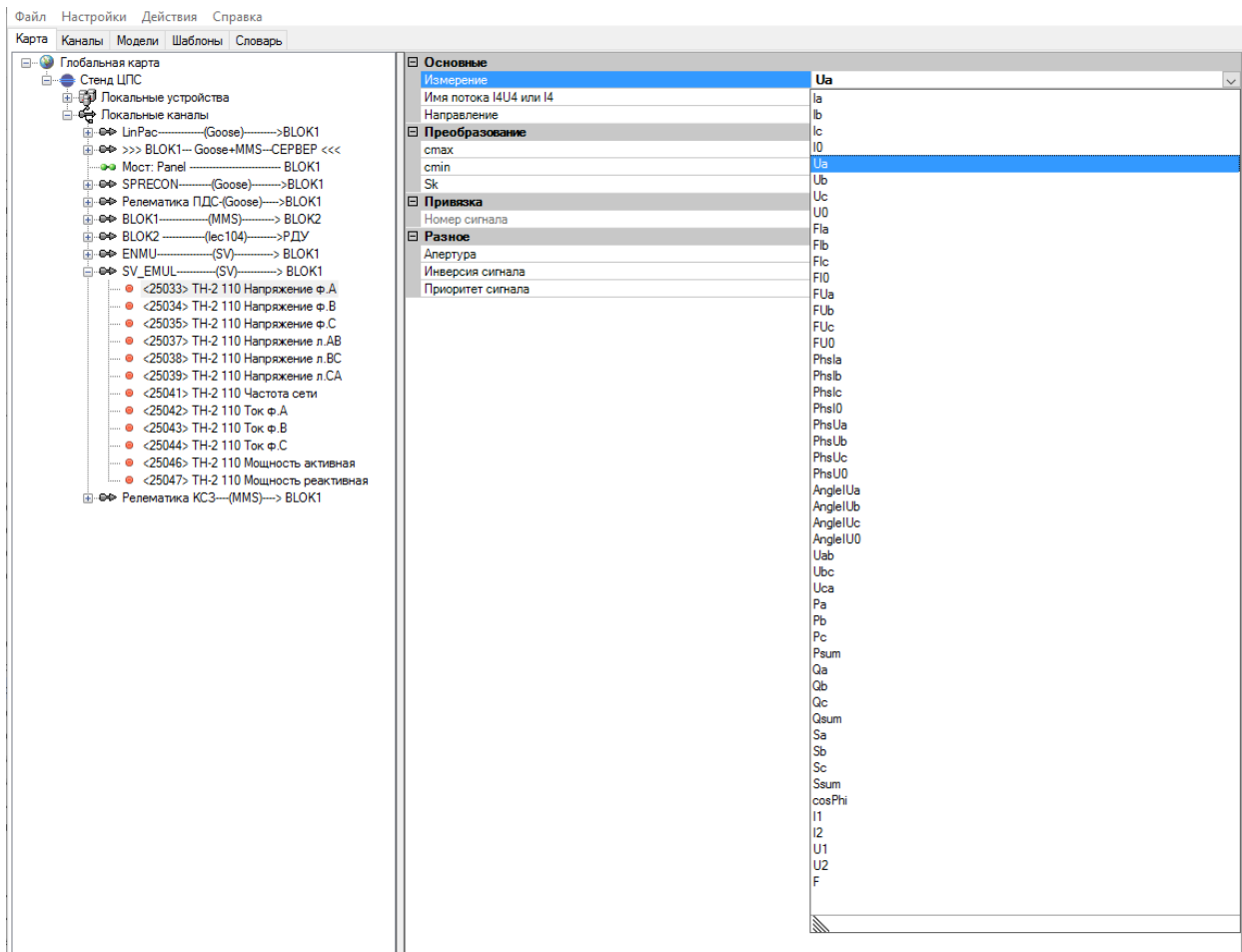
Рисунок 394. Настройка типа измерения в SV потоке
