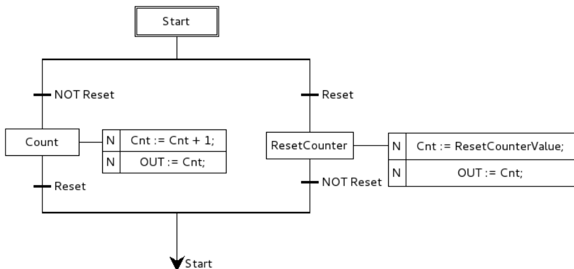
Рисунок 616. Смарт-Дизайнер ПЛК. Программа SFC. Альтернативное ветвление
