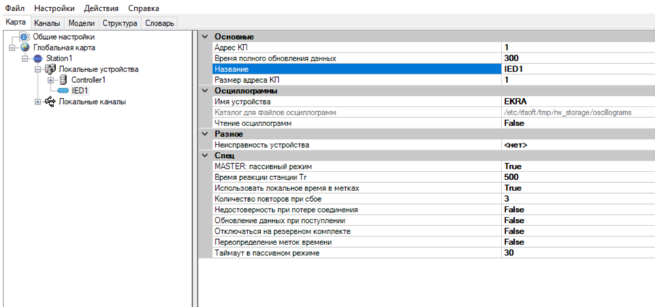
Рисунок 216. Настройка протокола с IED МЭК 60870-5-103
