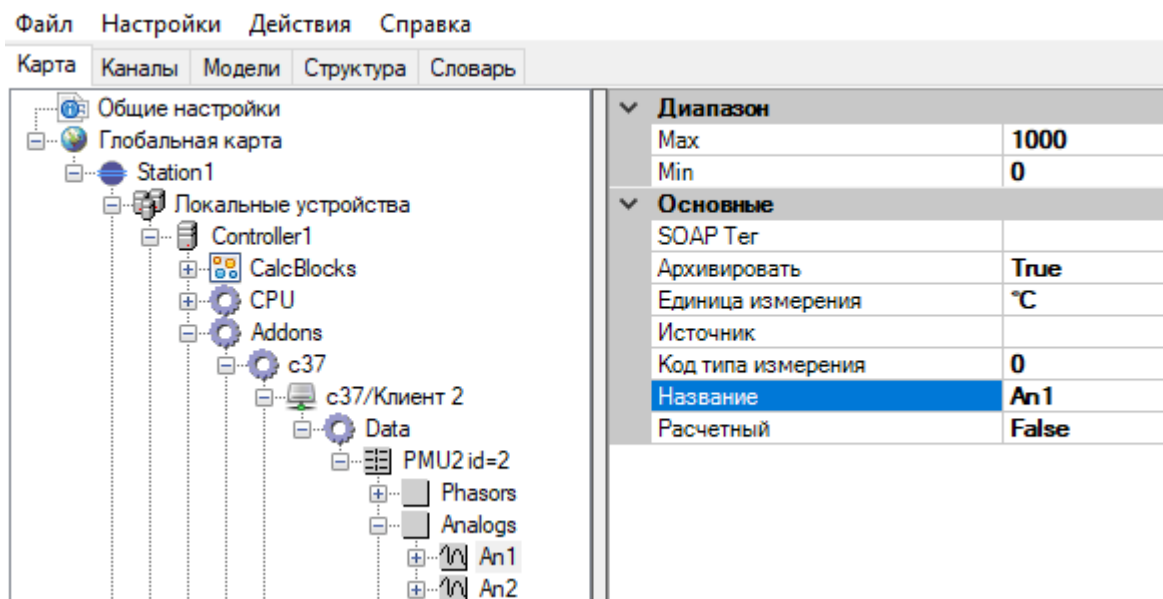
Рисунок 412. Настройка аналоговой величины
