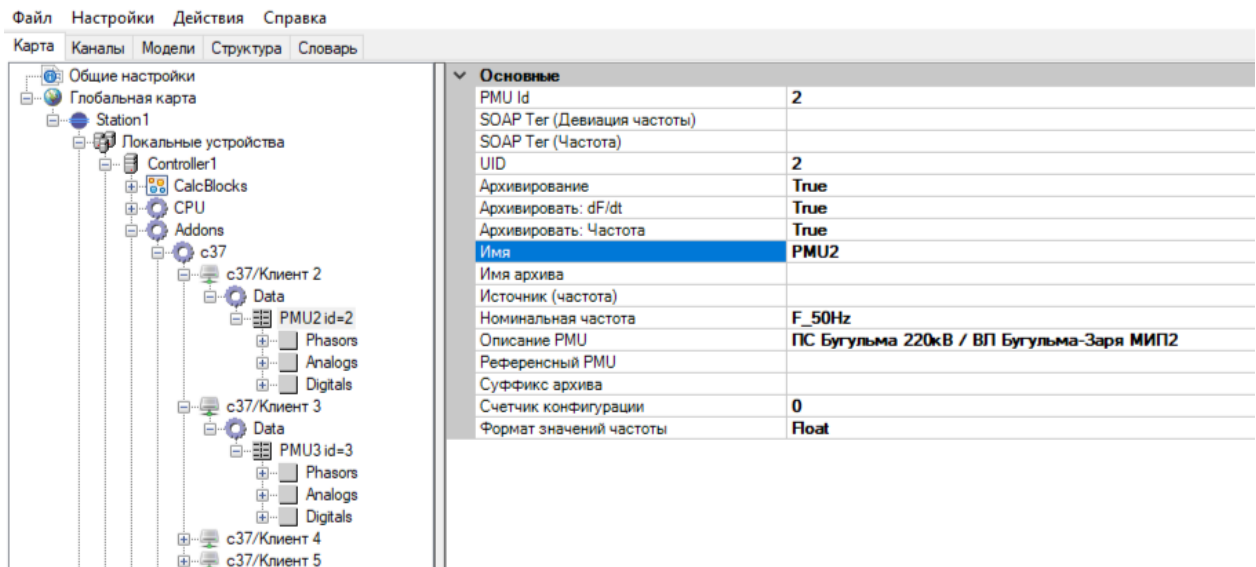
Рисунок 440. С37. Настройка архивирования dF/dt и частоты
