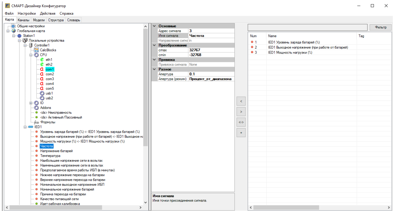
Рисунок 223. Привязка переменных в канале UPSLink
