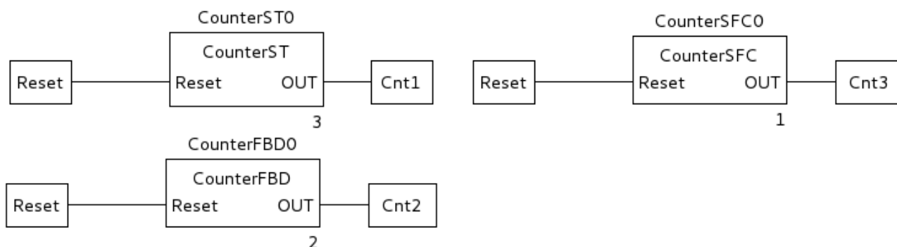
Рисунок 598. Смарт-Дизайнер ПЛК. Программа FBD. Схема с порядком выполнения заданным вручную
