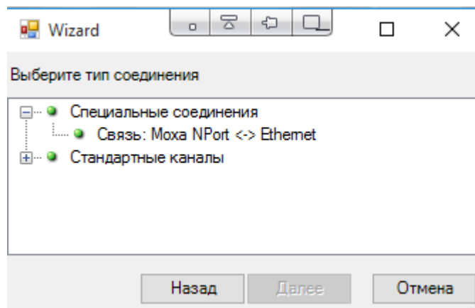
Рисунок 75. Подключение канального адаптера «Мохв NPort»
