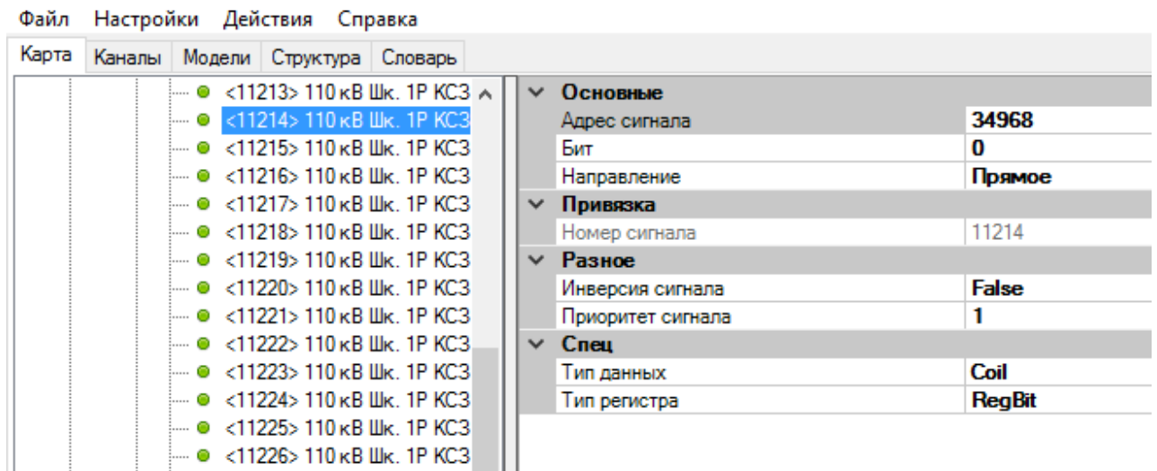
Рисунок 258. Настройки ТС в канале связи Modbus Uni/TCP
