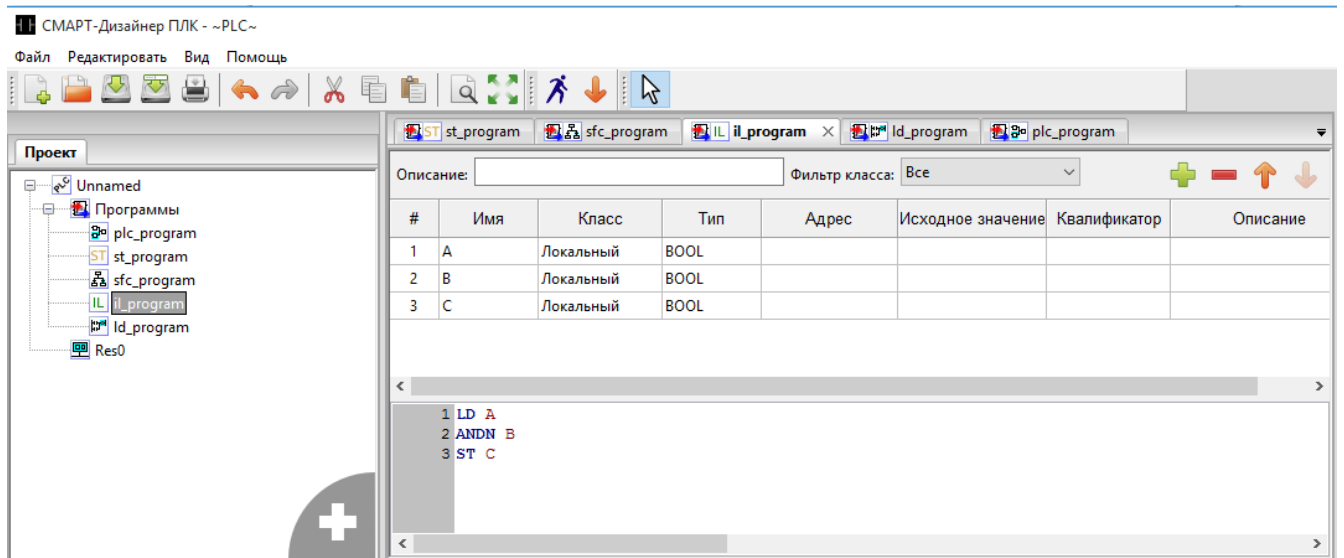
Рисунок 621. Смарт-Дизайнер ПЛК. Программа IL
