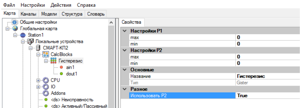
Рисунок 160. Функциональный блок Гистерезис
