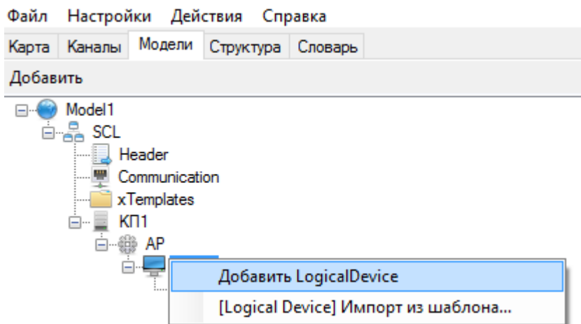
Рисунок 352. Объектная модель. Добавление логического устройства IED-устройства
