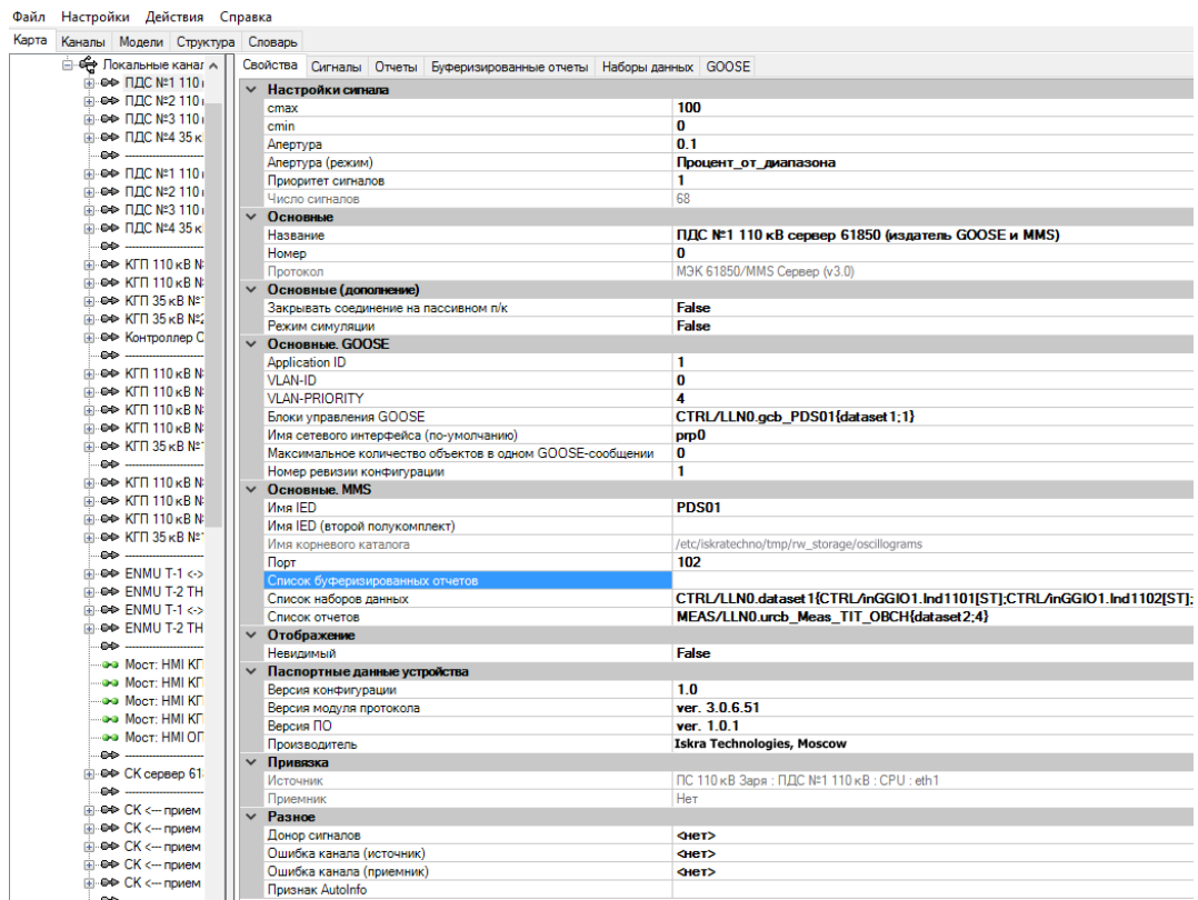
Рисунок 385. MMS сервер. Настройки канала связи
