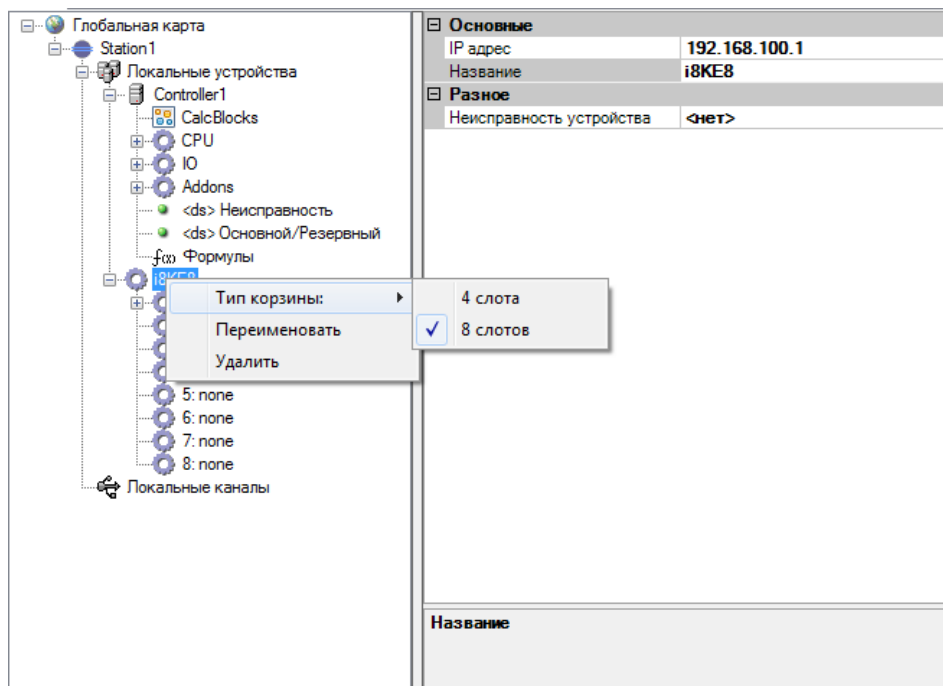
Рисунок 63. Результат подключения корзины расширения «i8KE8»
