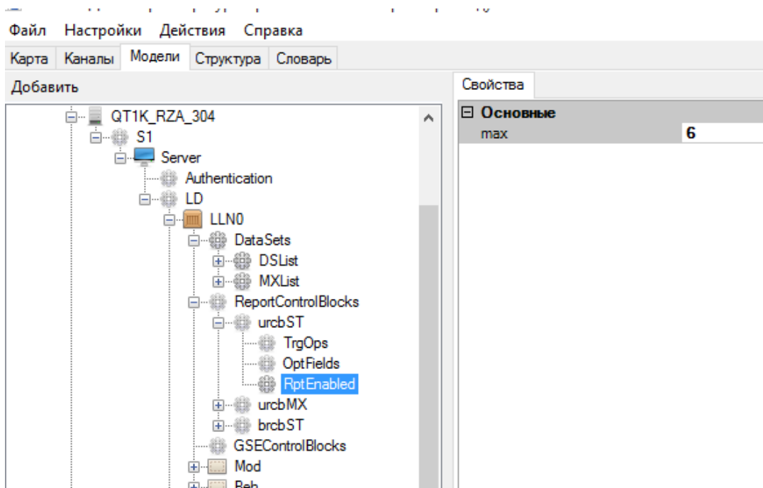
Рисунок 327. Объектная модель. Атрибут отчета RptEnabled
