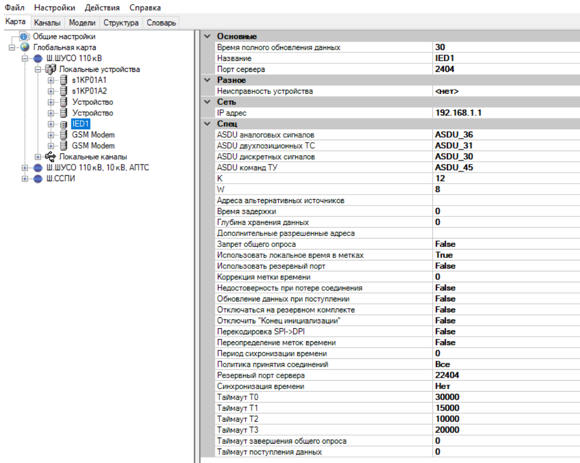
Рисунок 190. Настройка протокола передачи данных IED устройства
