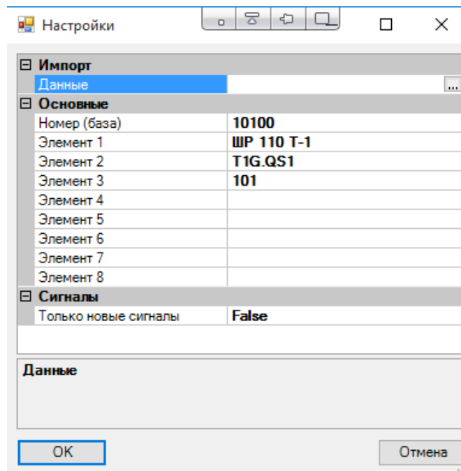
Рисунок 474. Автозаполнение полей формы импорта из структуры
