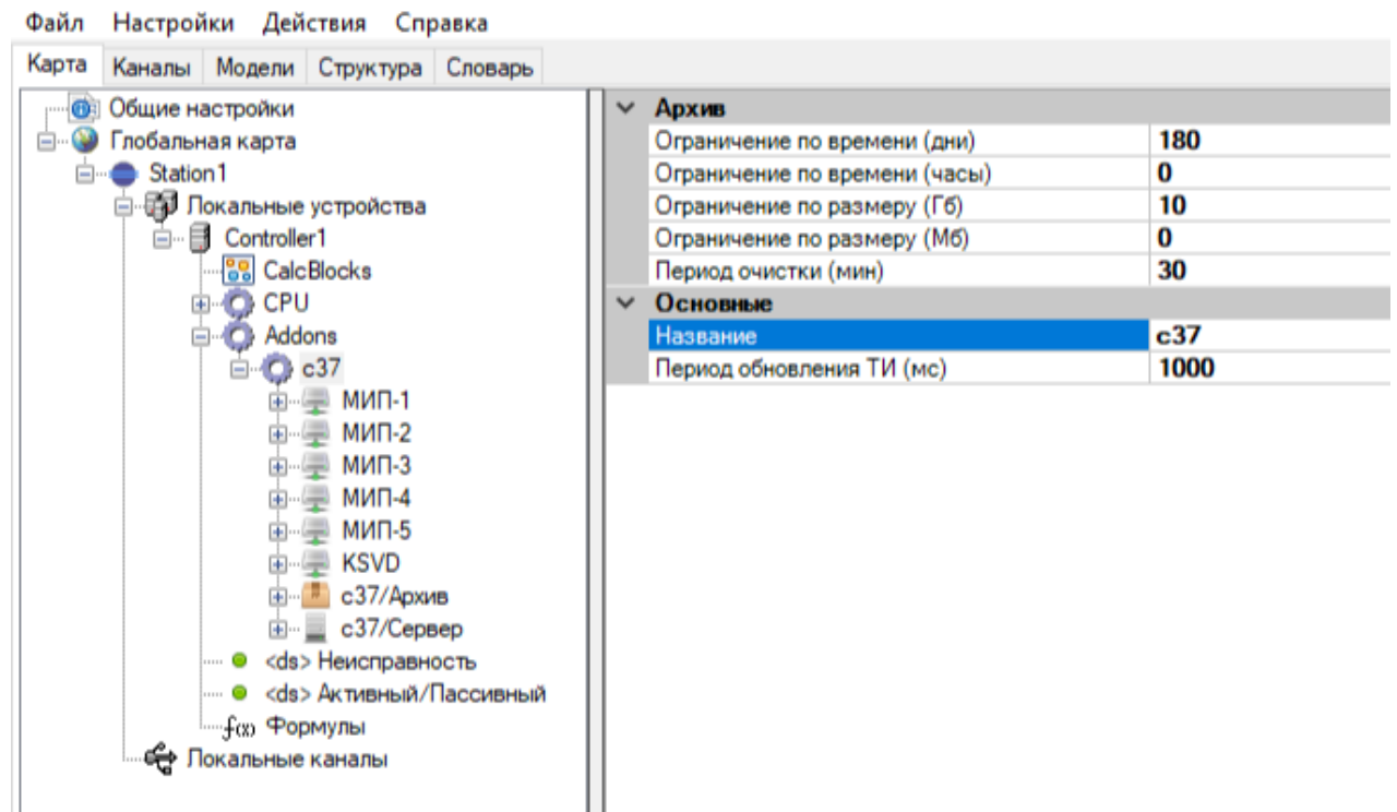
Рисунок 399. С37. Пример КСВД
