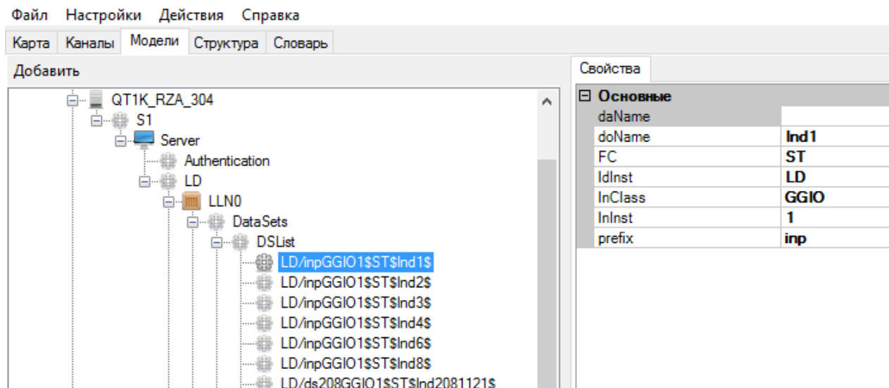
Рисунок 323. Объектная модель. Формирование набора данных
