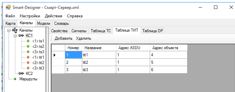
Рисунок 236. Вкладка «Таблица ТИТ»
