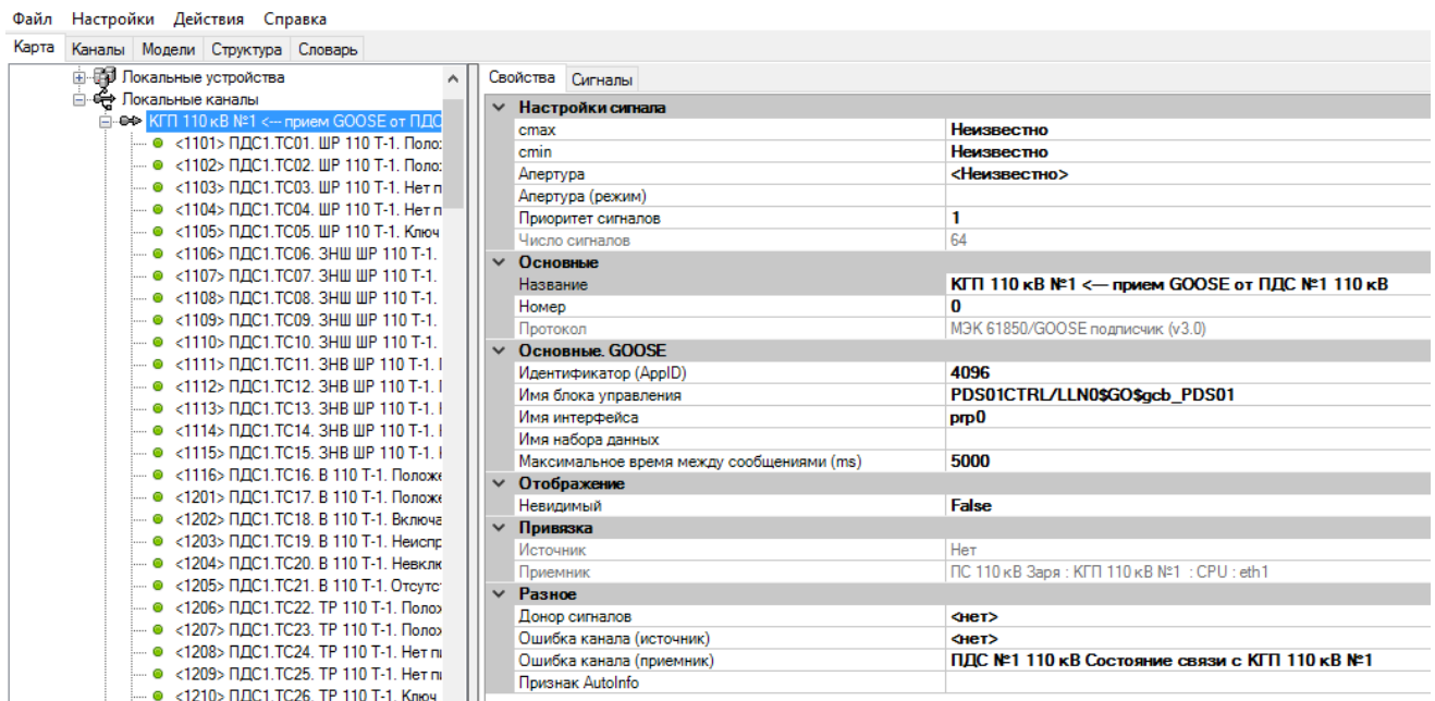
Рисунок 390. Пример настройки GOOSE
