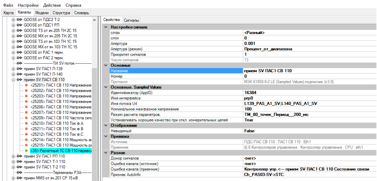
Рисунок 392. Пример настройки SV потоков
