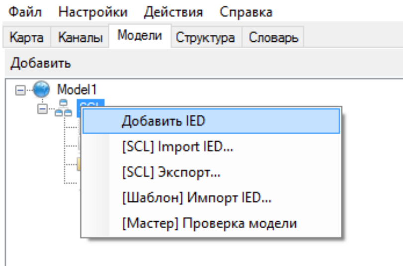
Рисунок 350. Объектная модель. Ручное добавление IED-устройства
