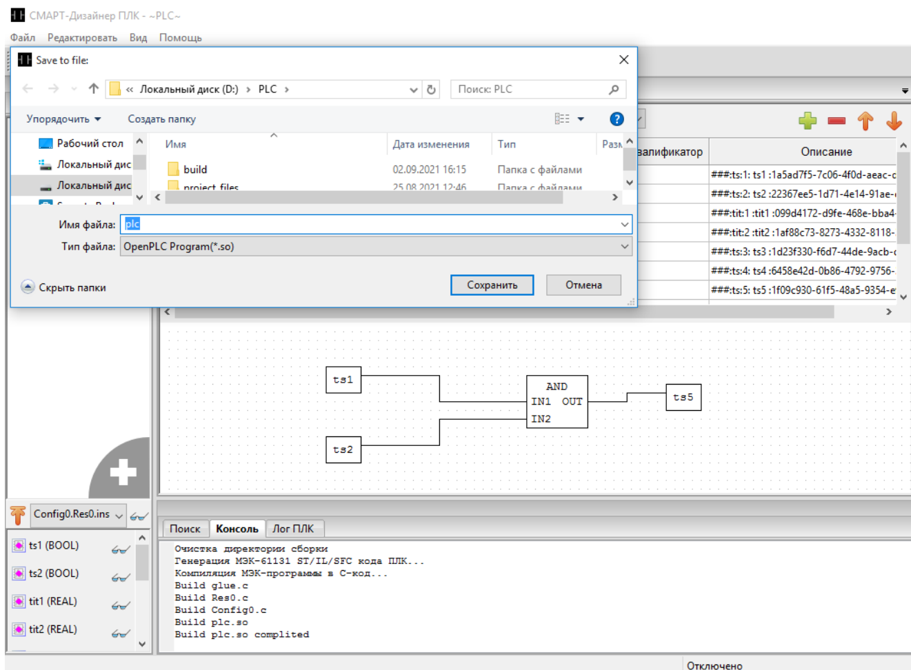
Рисунок 624. Смарт-Дизайнер ПЛК. Компиляция проекта
