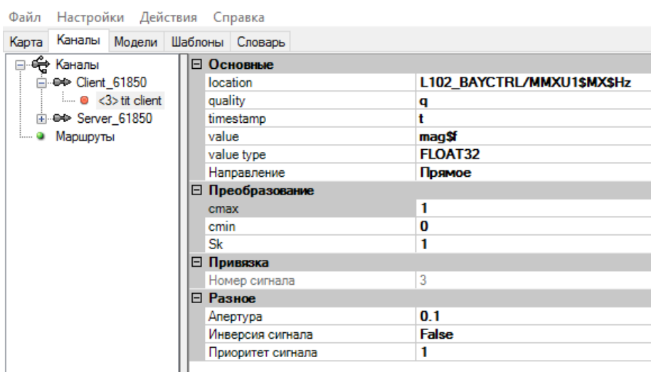
Рисунок 383. MMS клиент. Настройки переменных
