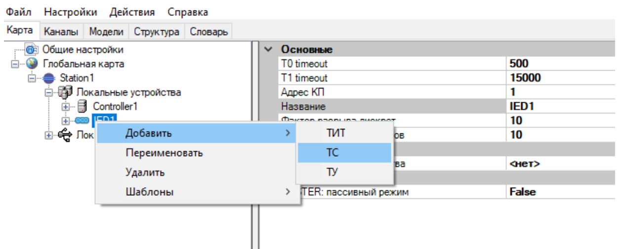
Рисунок 204. Добавление переменных в IED Modbus TCP
