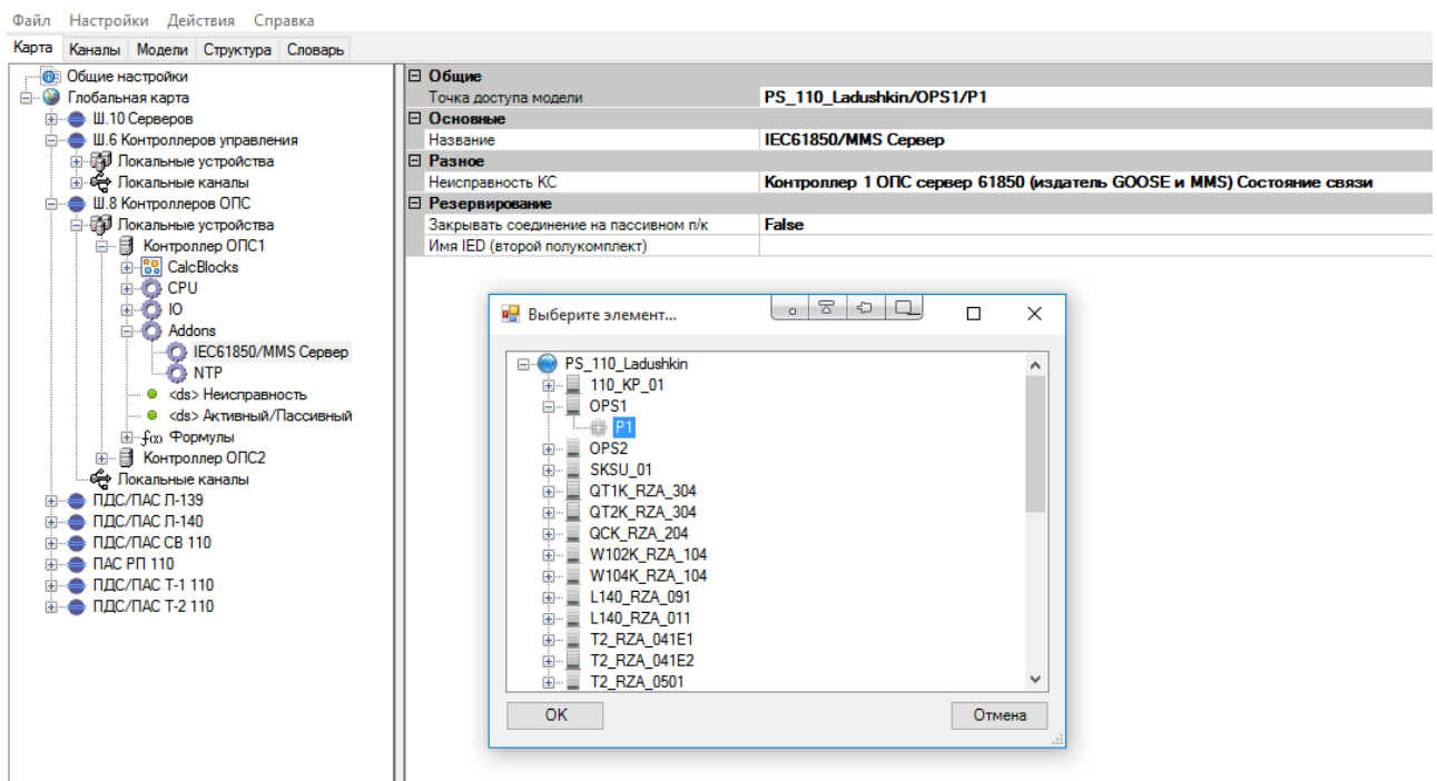
Рисунок 336. MMS сервер. Создание ссылки на отчет
