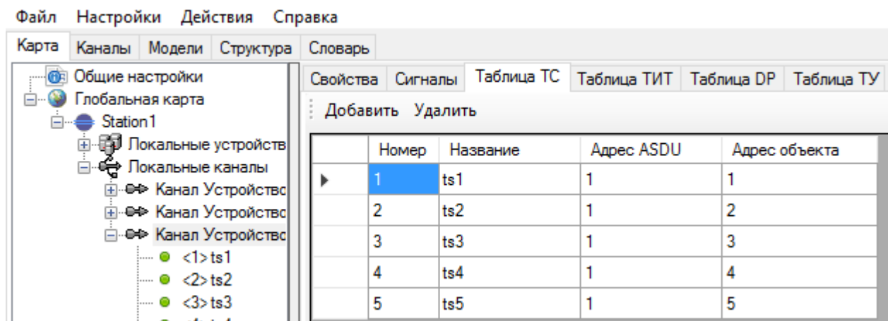
Рисунок 252. Настройки адресации переменных канала связи МЭК60870-5-104
