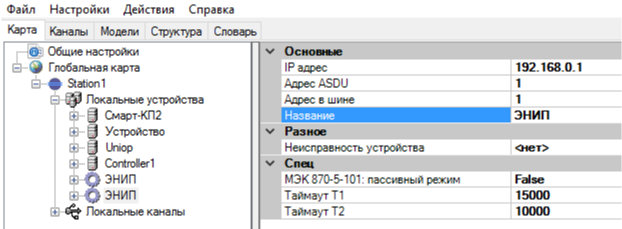
Рисунок 168. Конфигурирование устройства «ЭНИП»
