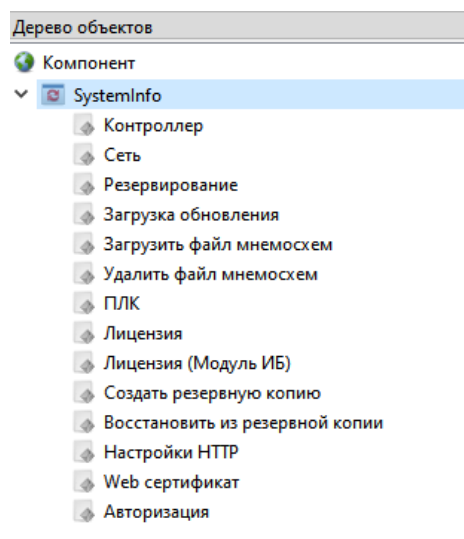
Рисунок 513. Список опций параметрирования устройства
