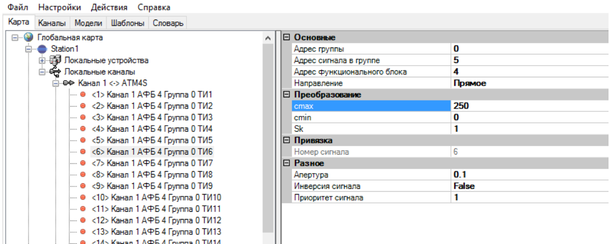
Рисунок 296. Настройки ТИ канала связи Гранит
