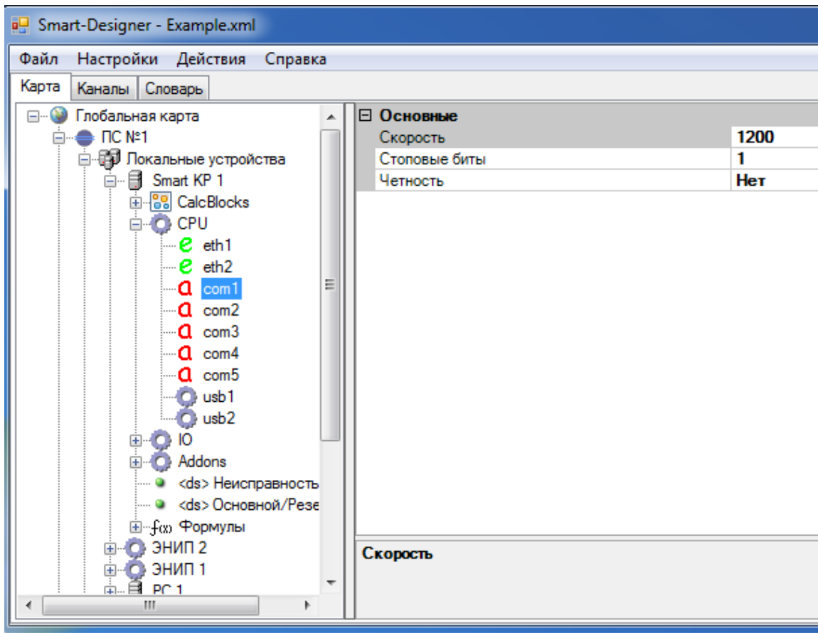
Рисунок 70. Конфигурирование канального адаптера «АТМ4»
