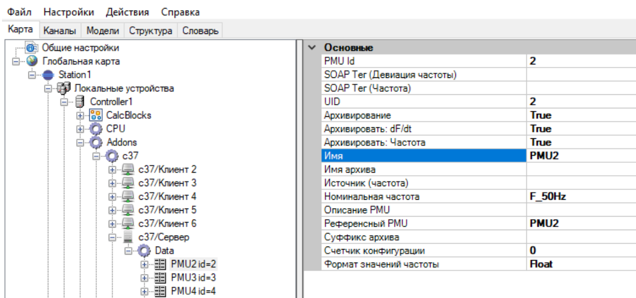
Рисунок 436. С37. Настройка УСВИ
