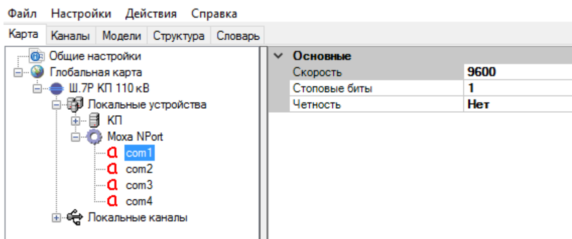
Рисунок 78. Конфигурирование портов канального адаптера «Мохха NPort»
