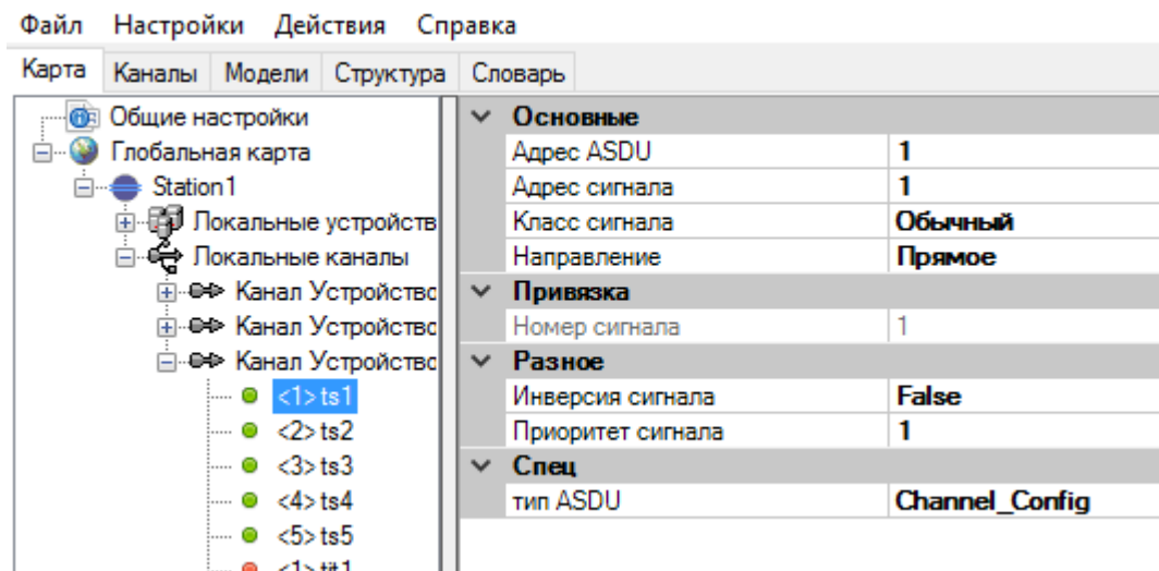
Рисунок 251. Настройки переменных канала связи МЭК60870-5-104
