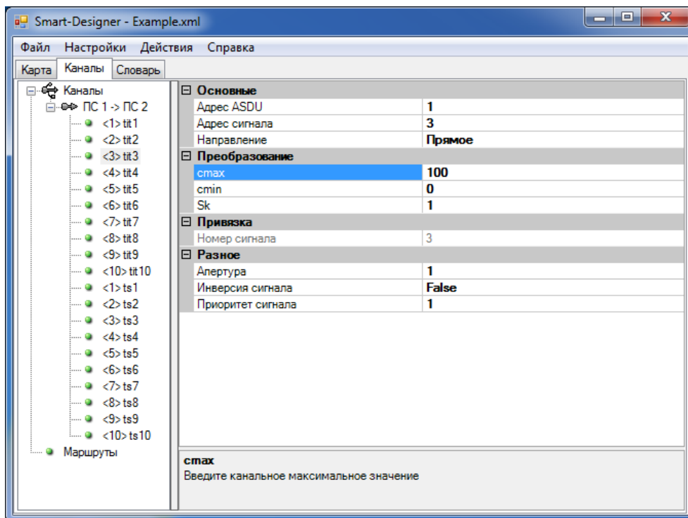
Рисунок 234. Работа с переменными канала передачи данных
