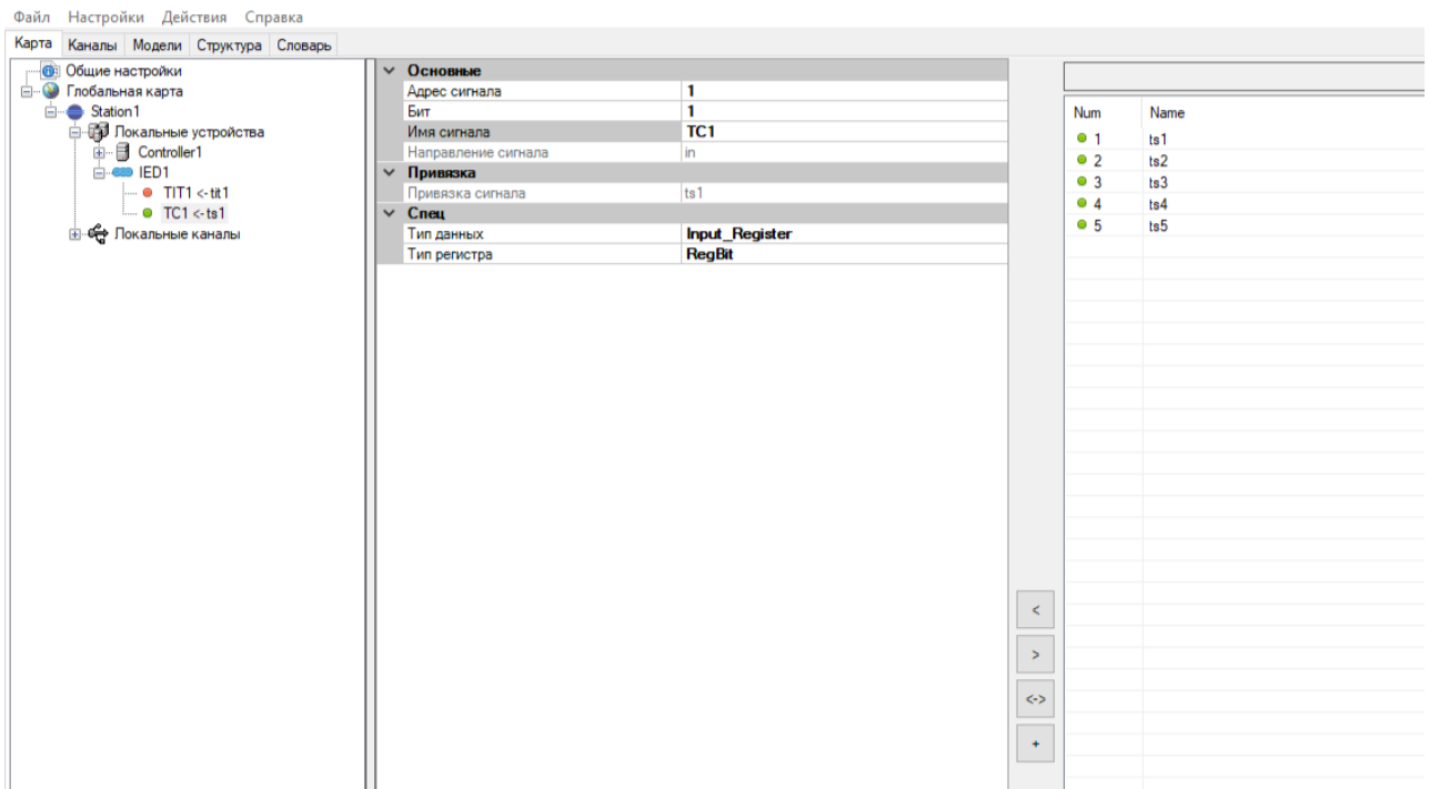
Рисунок 199. Привязка переменных к IED Modbus RTU
