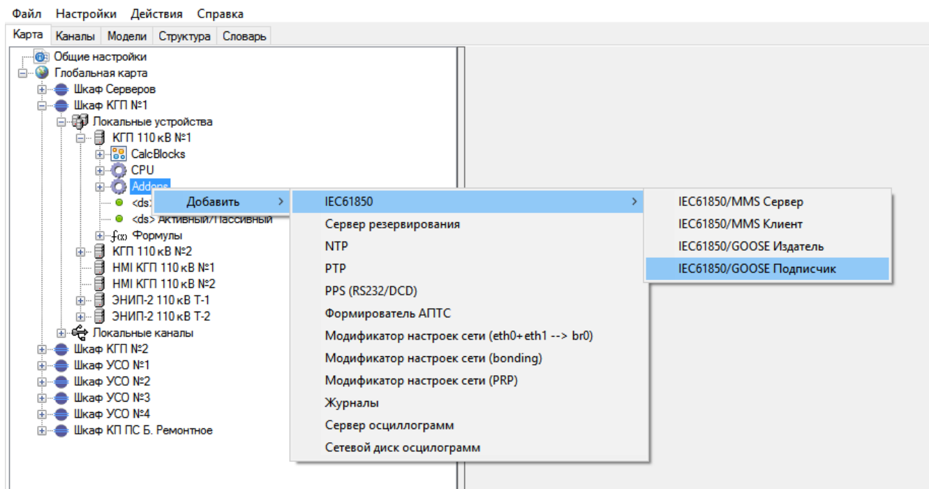
Рисунок 337. Добавление GOOSE подписчика
