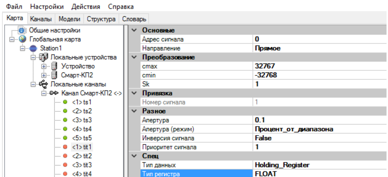
Рисунок 259. Настройки ТИ в канале связи Modbus Uni/TCP
