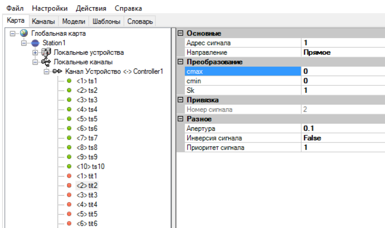
Рисунок 300. Настройки ТИ канала связи КАРС-ТП
