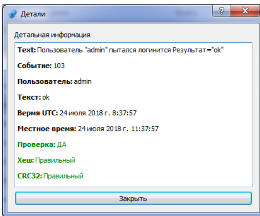
Рисунок 577. Загруженный журнал безопасности
