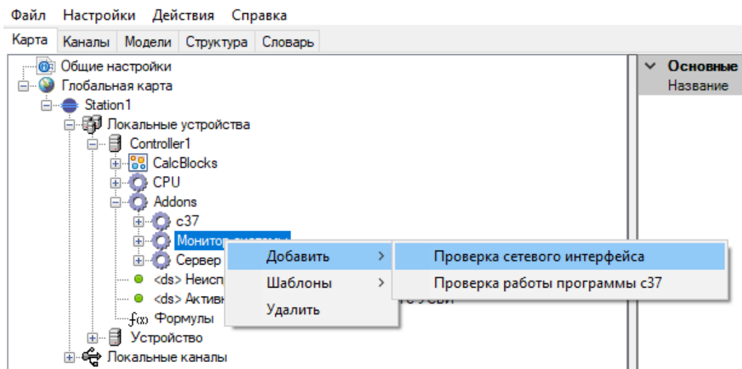
Рисунок 118. Добавление проверки сетевого интерфейса
