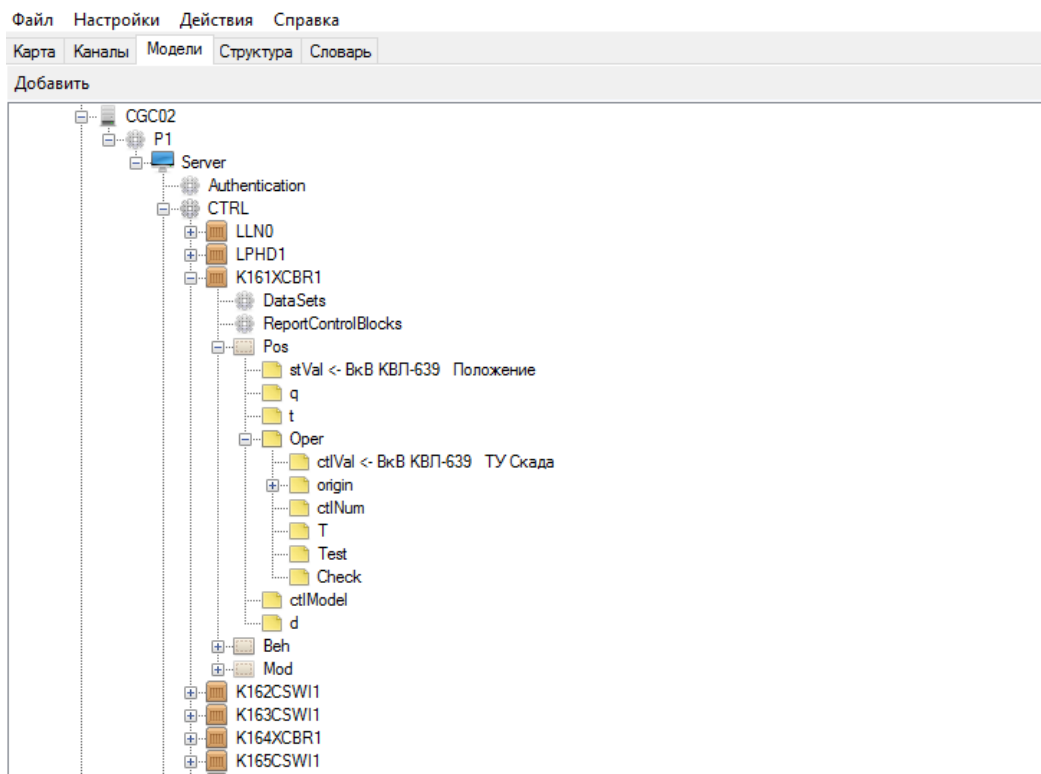
Рисунок 355. Объектная модель. Добавление логического узла коммутационного аппарата
