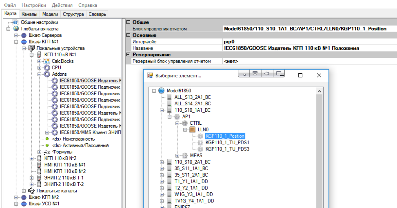
Рисунок 342. GOOSE издатель. Создание ссылки на блок управления
