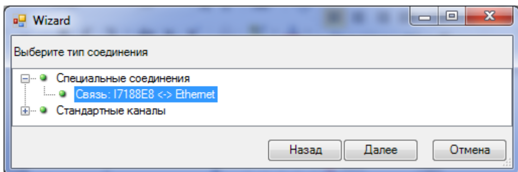
Рисунок 71. Подключение канального адаптера «I-7188E8»
