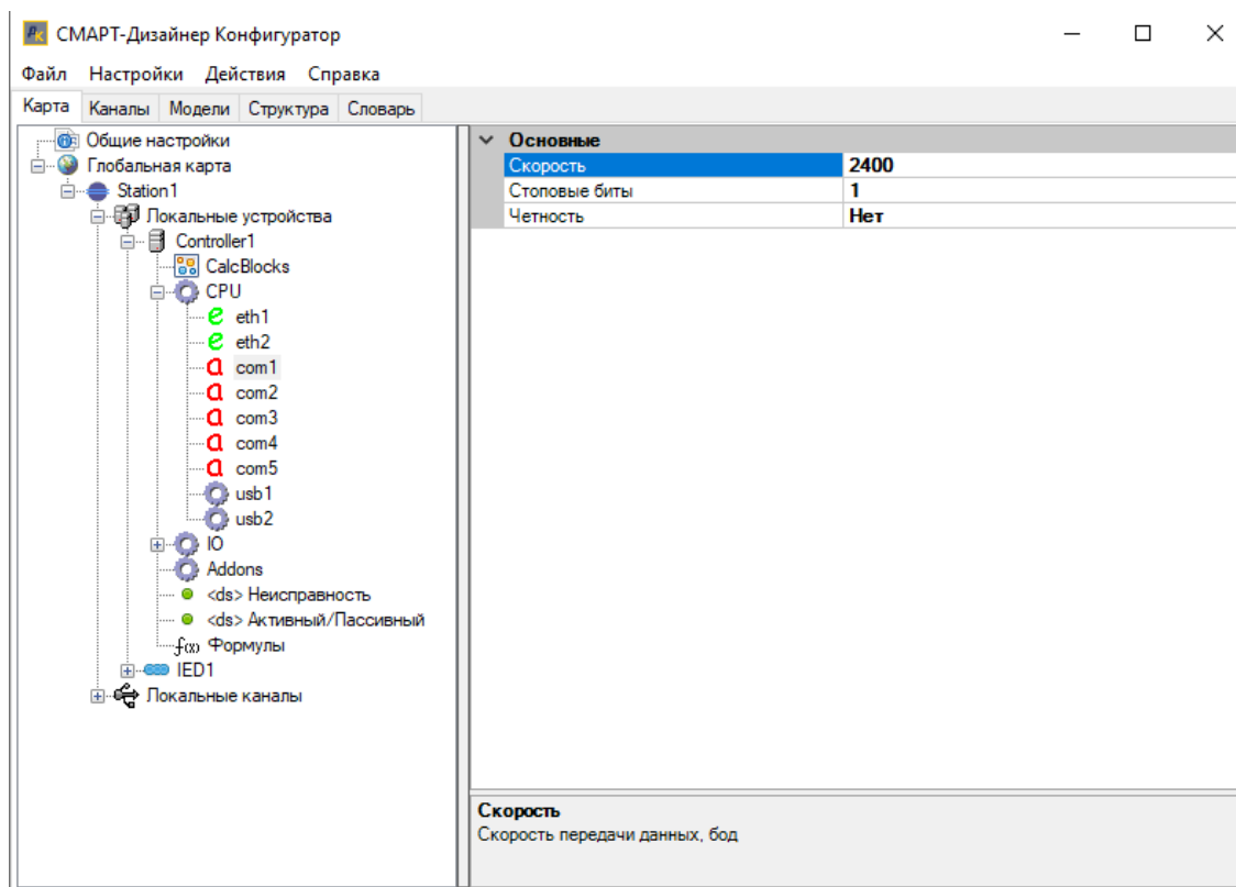
Рисунок 196. Настройка порта на контроллере для связи с IED Modbus RTU
