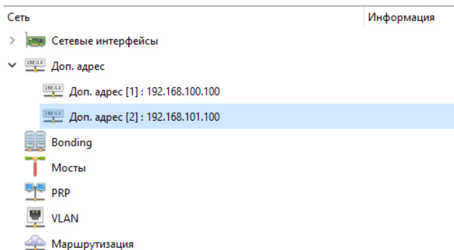
Рисунок 539. Узел «Доп. адрес»
