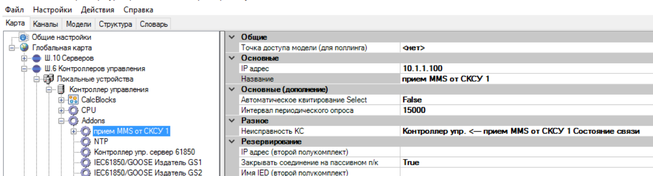
Рисунок 330. Настройка MMS клиента
