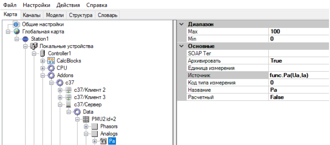
Рисунок 434. С37. Пример расчета активной мощности фазы А
