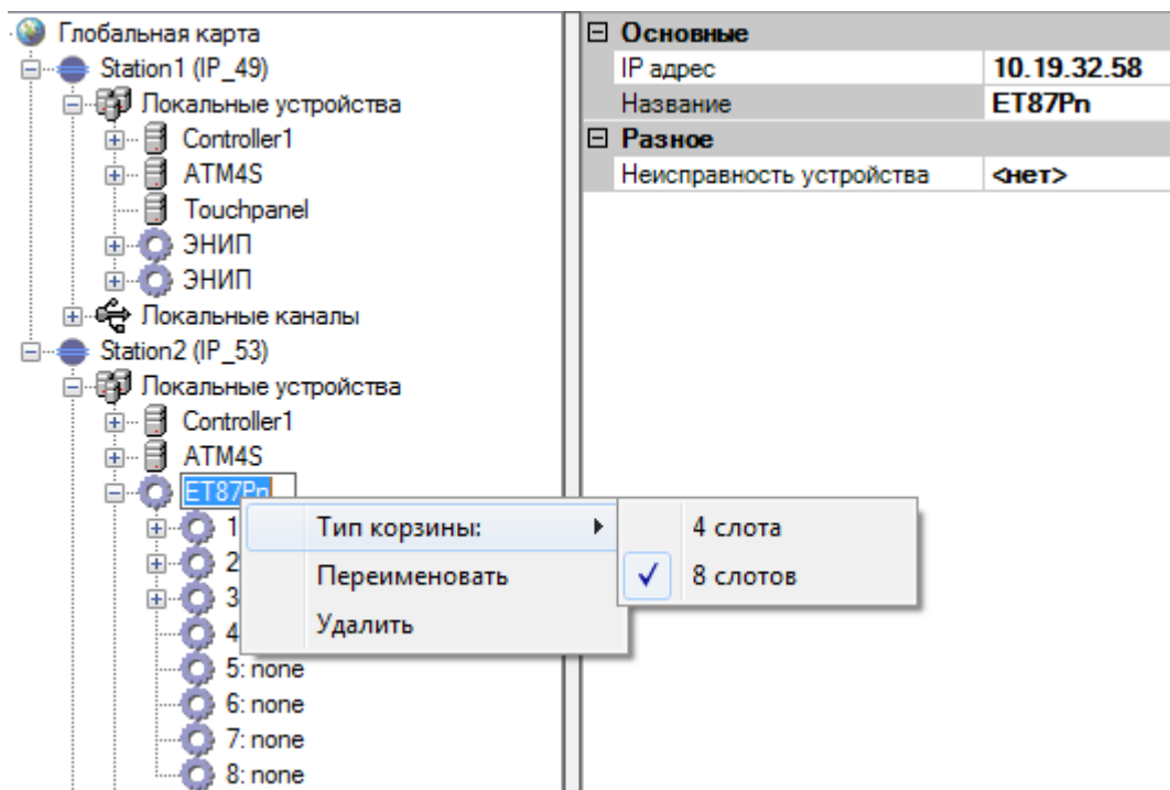
Рисунок 55. Результат подключения корзины расширения «ET-87Pn»
