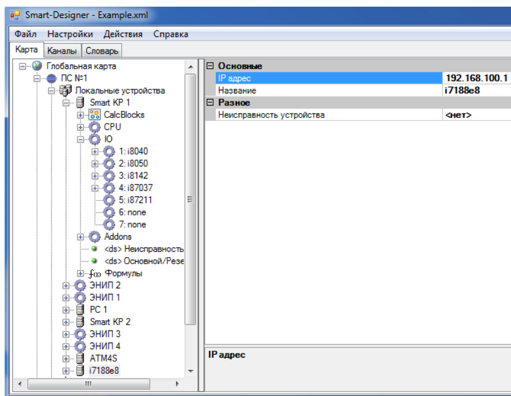
Рисунок 73. Конфигурирования канального адаптера «I-7188E8»
