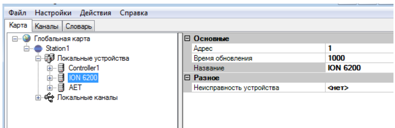
Рисунок 180. Конфигурирование устройства «ION»
