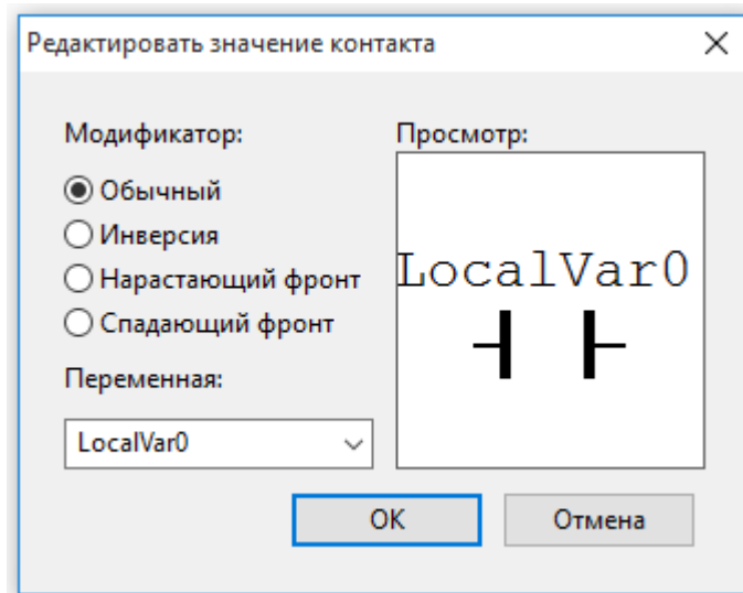
Рисунок 605. Смарт-Дизайнер ПЛК. Программа LD. Добавление контакта
