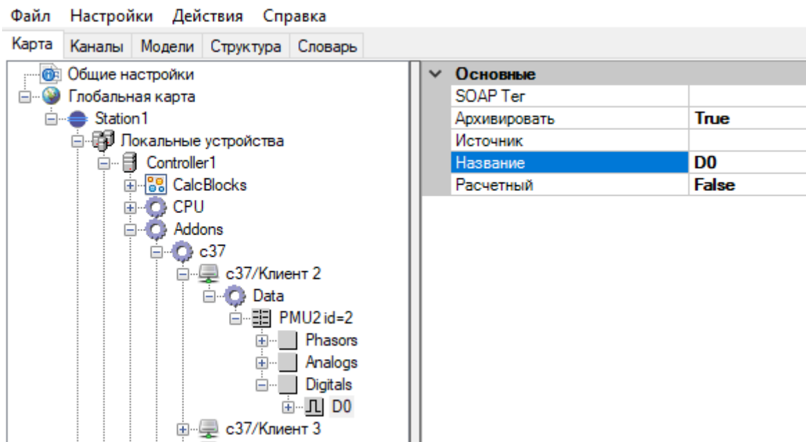
Рисунок 414. Настройка дискретной величины
