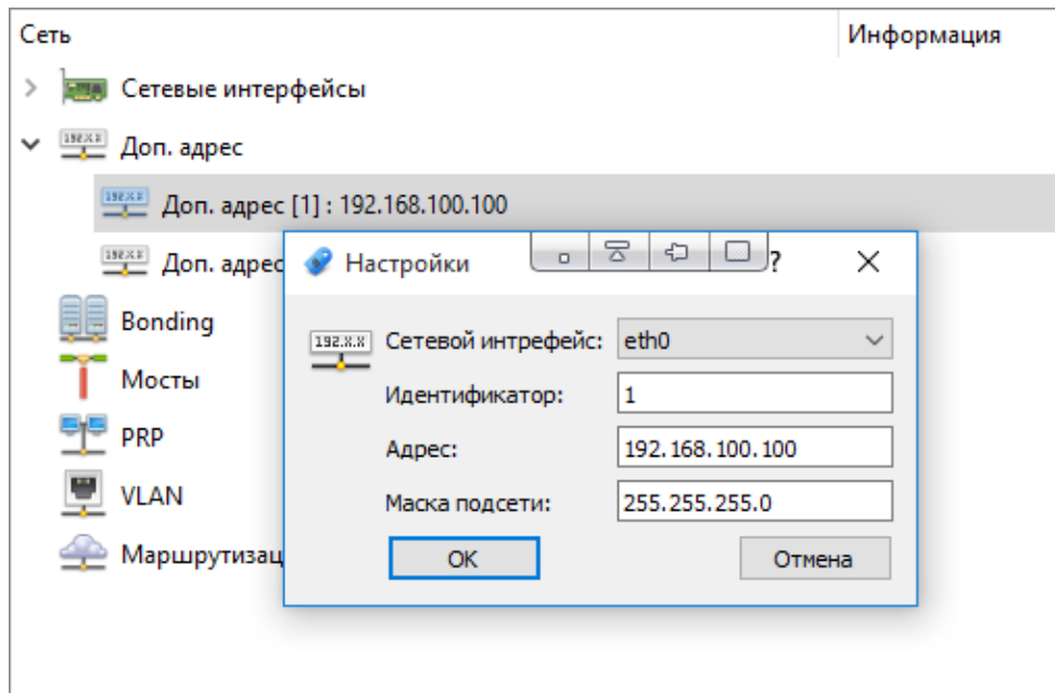
Рисунок 540. Настройка параметров дополнительных адресов
