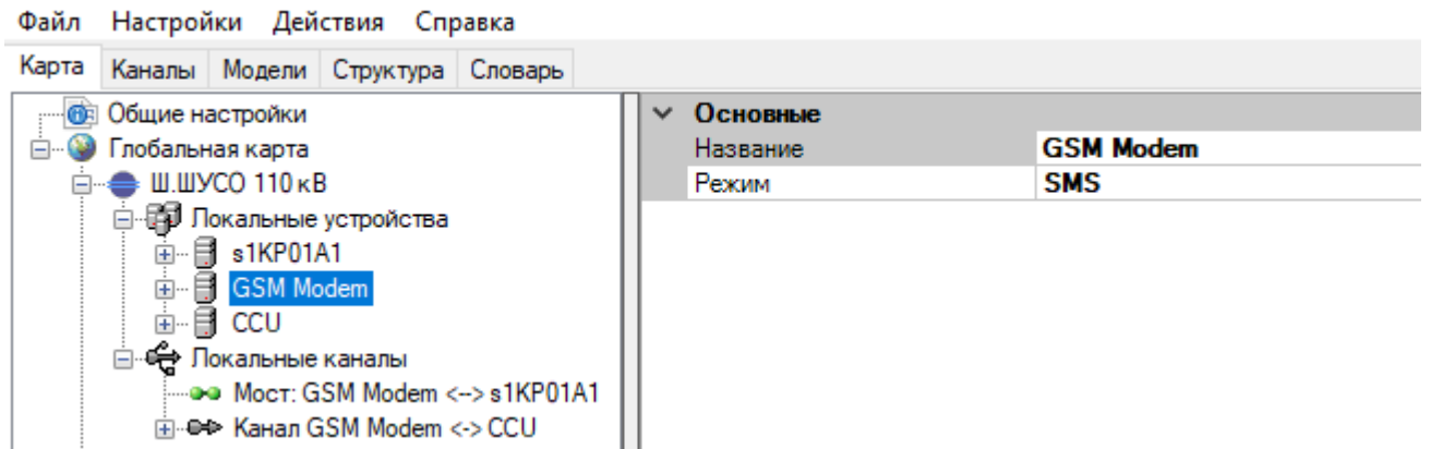
Рисунок 182. Конфигурирование модема для обмена СМС сообщениями
