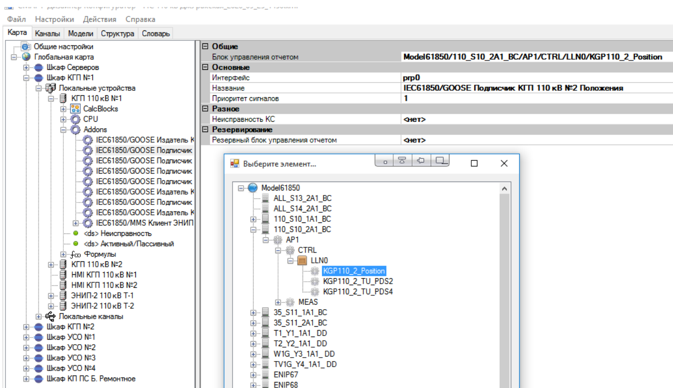
Рисунок 339. GOOSE подписчик. Создание ссылки на блок управления
