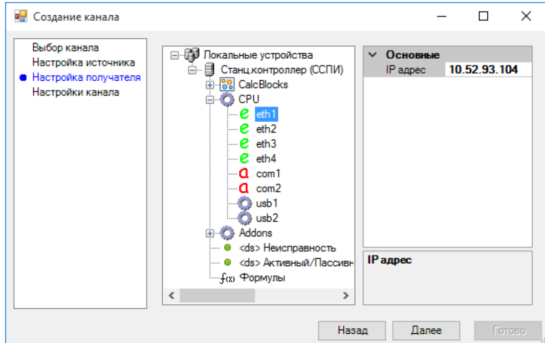
Рисунок 227. Выбор устройства приемника
