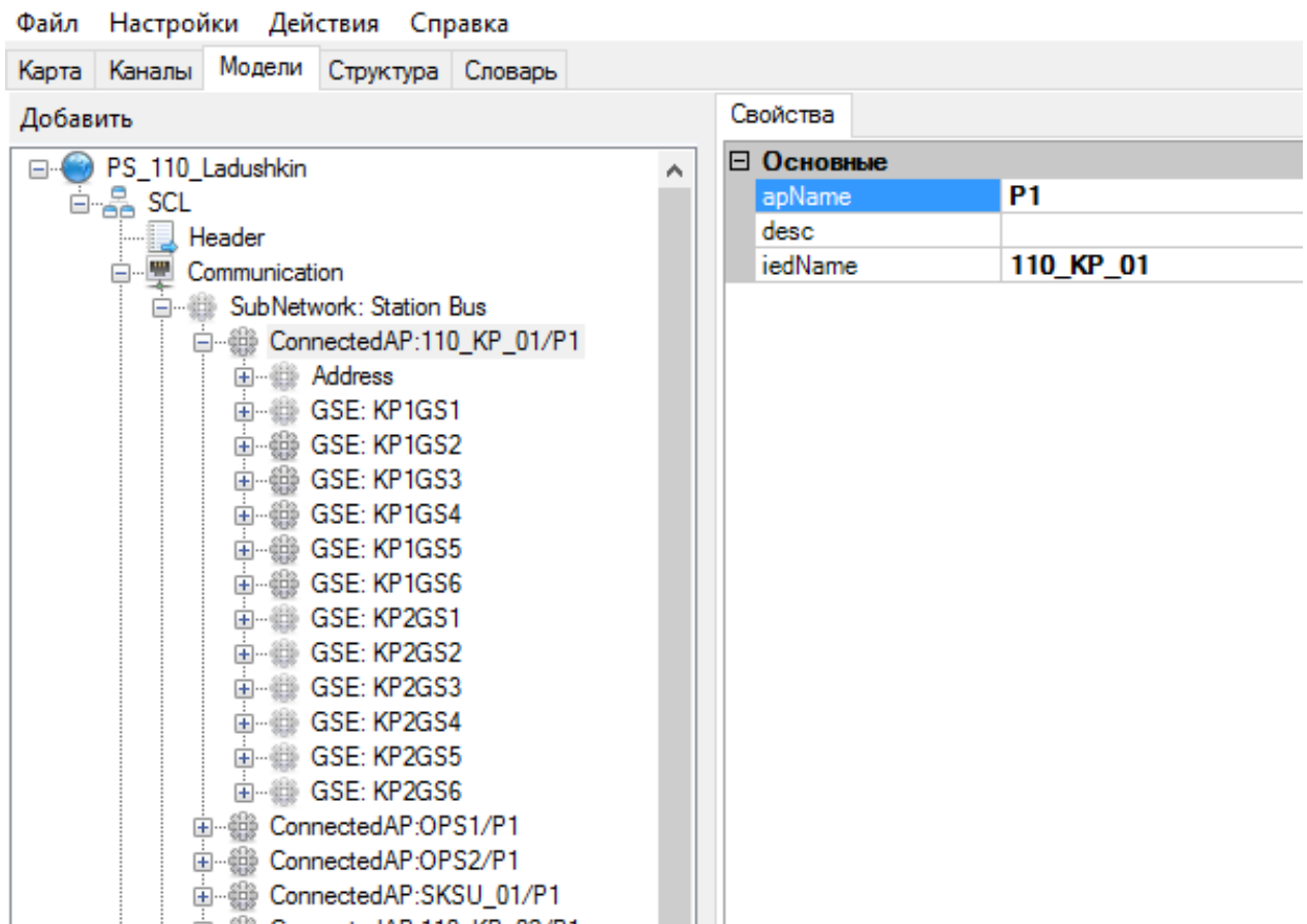
Рисунок 307. Объектная модель. Точка доступа к соединению (ConnectedAP)
