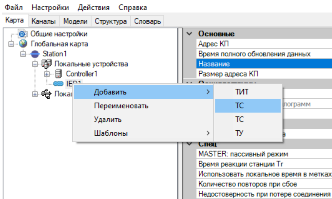
Рисунок 217. Добавление переменных в IED МЭК 60870-5-103
