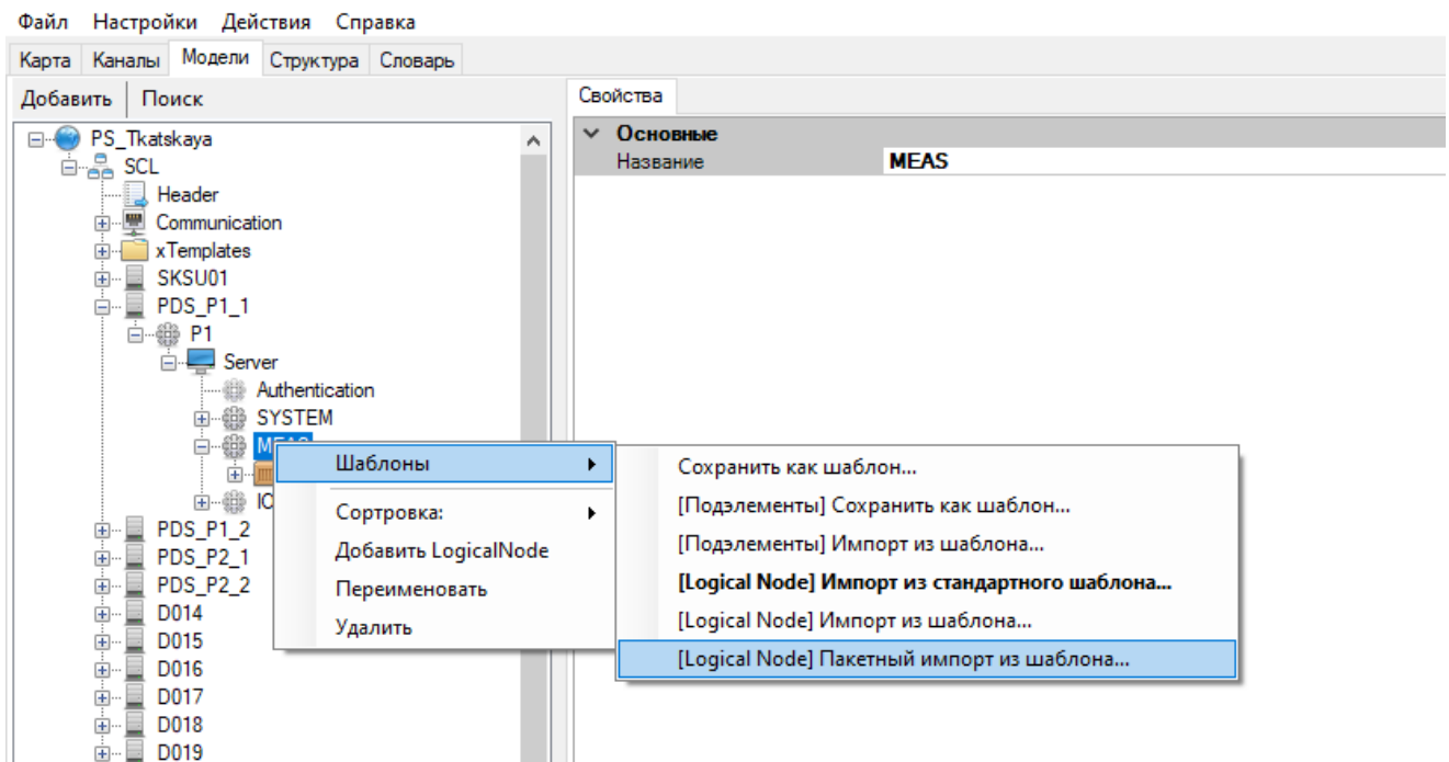
Рисунок 479. Пакетный импорт логических узлов из шаблона
