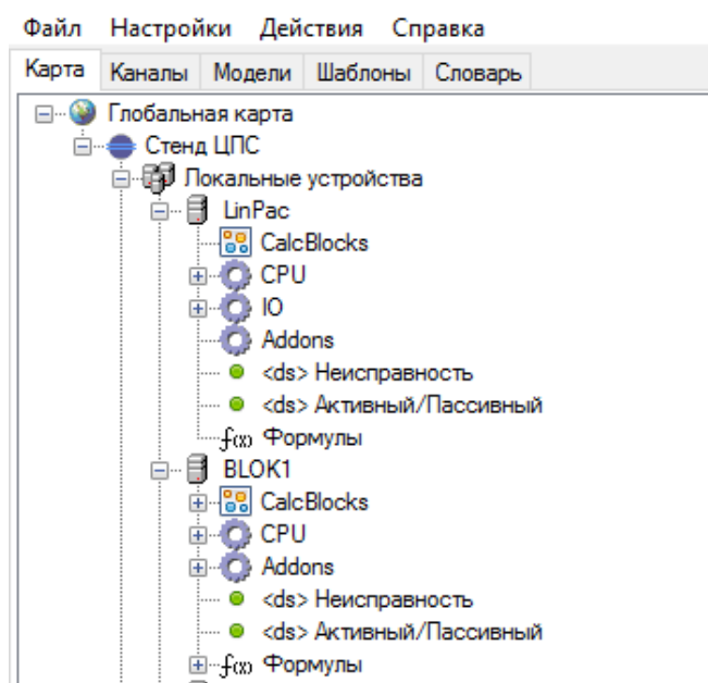
Рисунок 46. Структура контроллера
