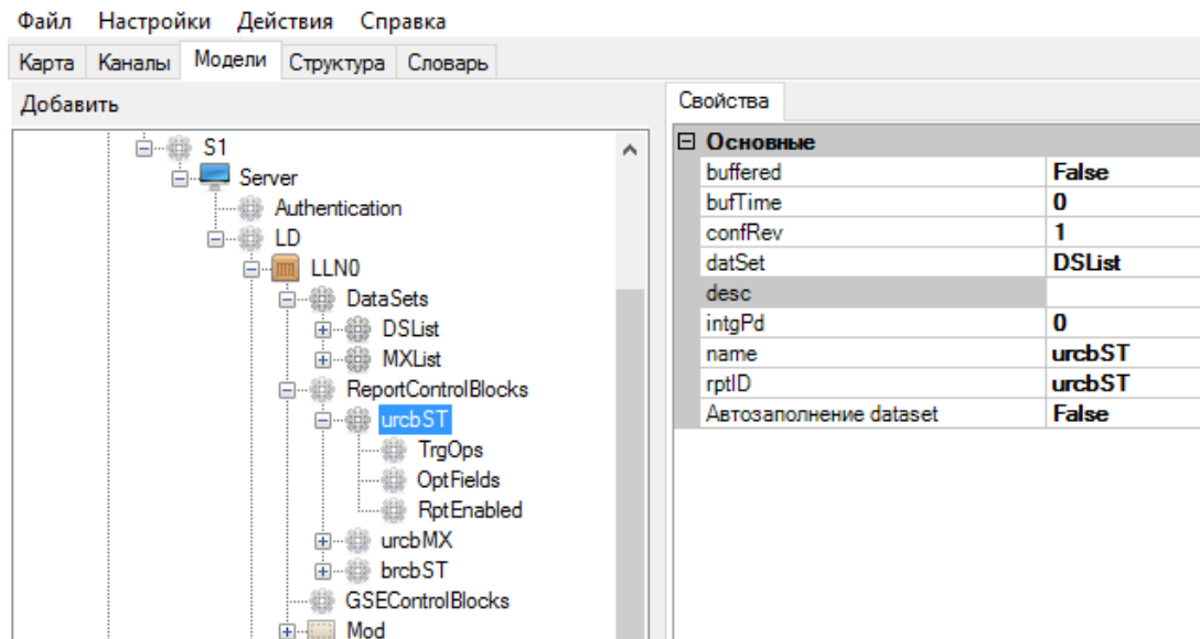
Рисунок 324. Объектная модель. Блок управления отчетами
