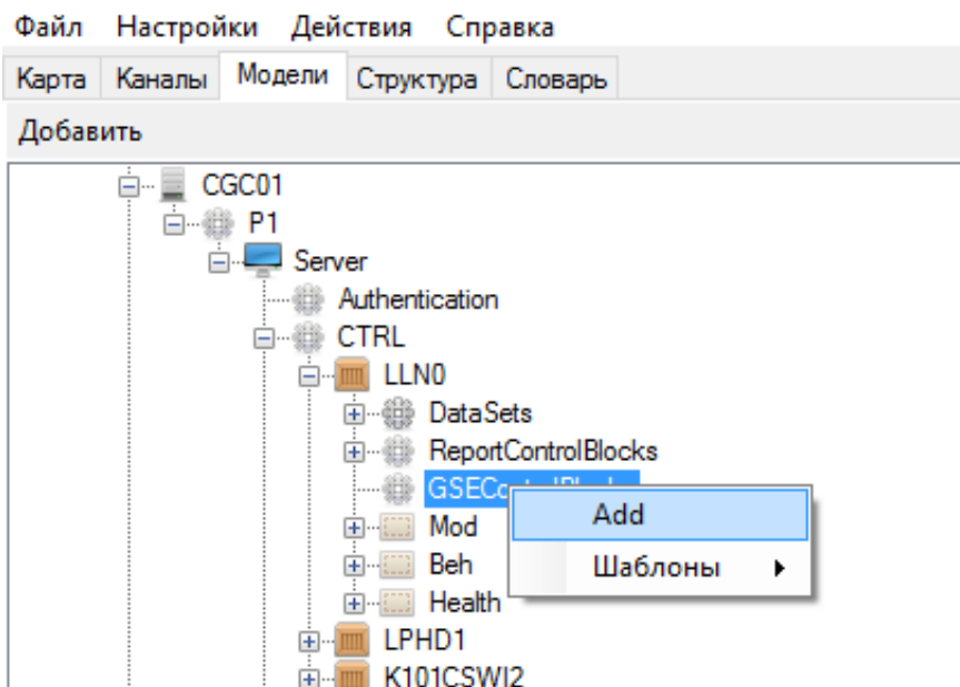
Рисунок 367. Объектная модель. Добавление блока управления GOOSE сообщениями
