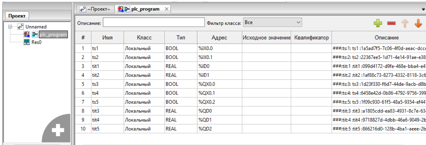
Рисунок 590. Smart-Дизайнер ПЛК. Переменные программы
