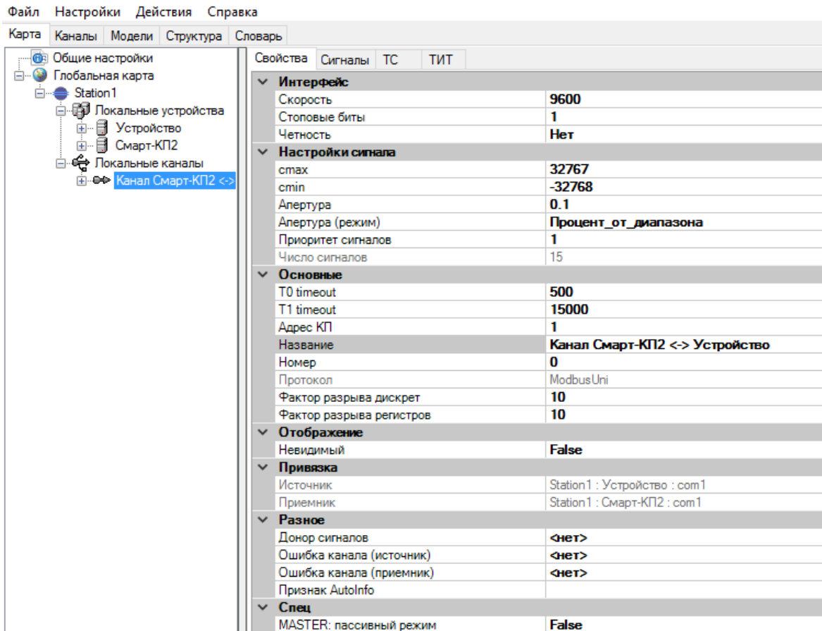
Рисунок 256. Настройки канала связи Modbus Uni
