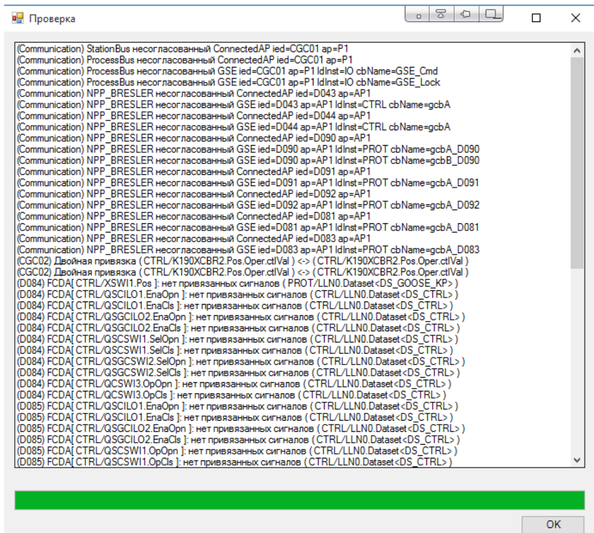
Рисунок 380. Объектная модель. Результат проверки модели
