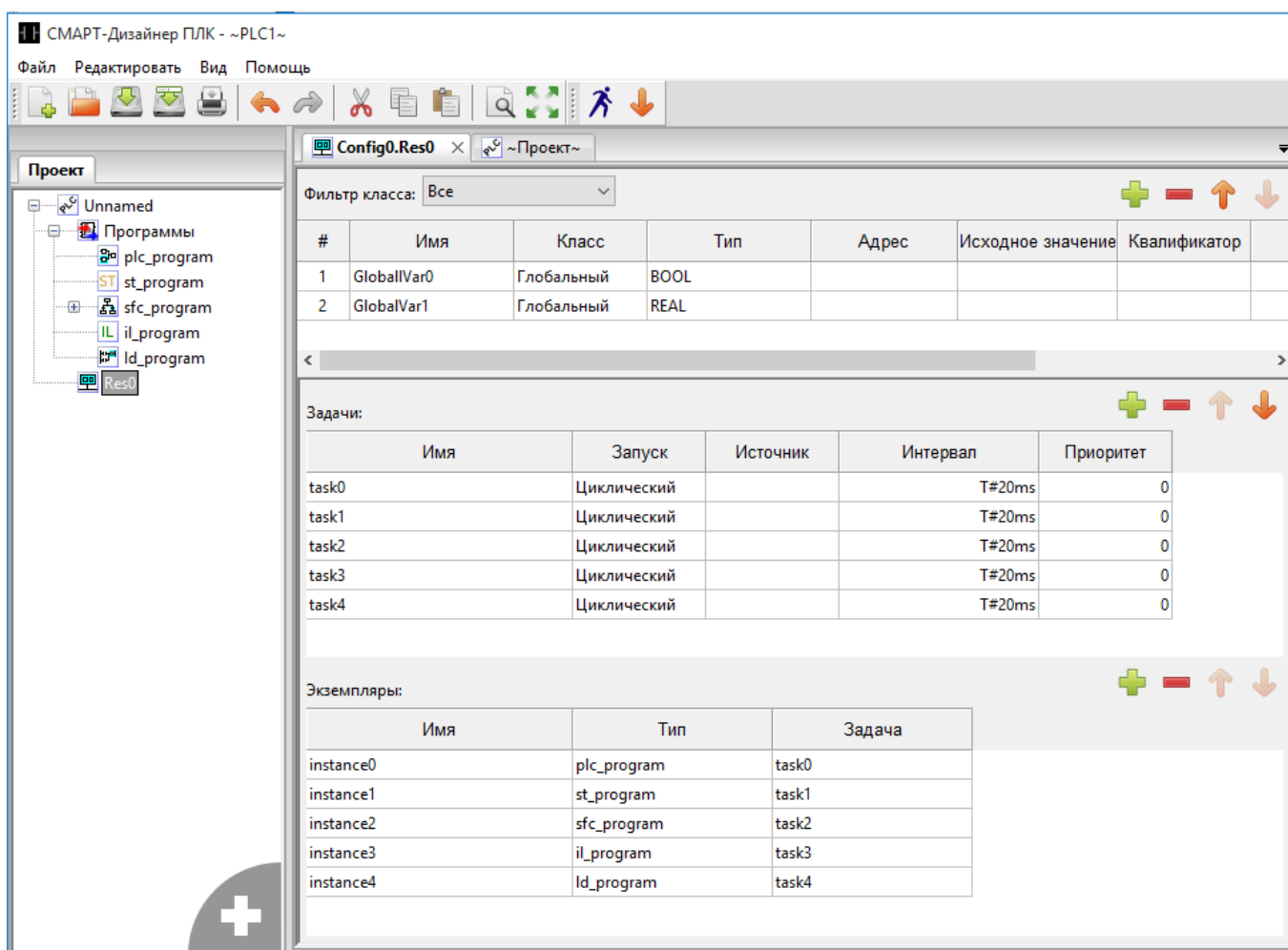
Рисунок 622. Смарт-Дизайнер ПЛК. Ресурс проекта
