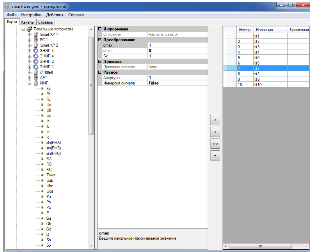
Рисунок 177. Привязка переменных к устройству «МИП»
