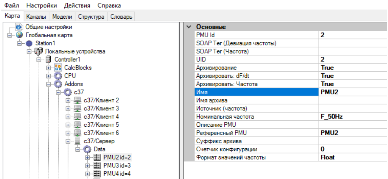
Рисунок 422. С37. Настройка УСВИ
