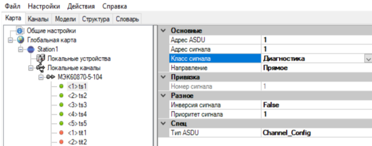
Рисунок 253. Настройка диагностических переменных канала связи МЭК60870-5-104
