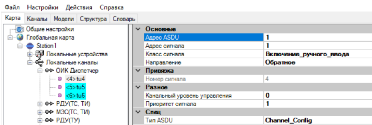
Рисунок 254. Прием команды установки ручного ввода из ОИК Диспетчер
