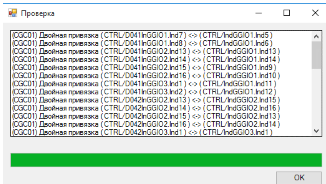
Рисунок 377. Объектная модель. Результат проверки привязок в IED устройстве
