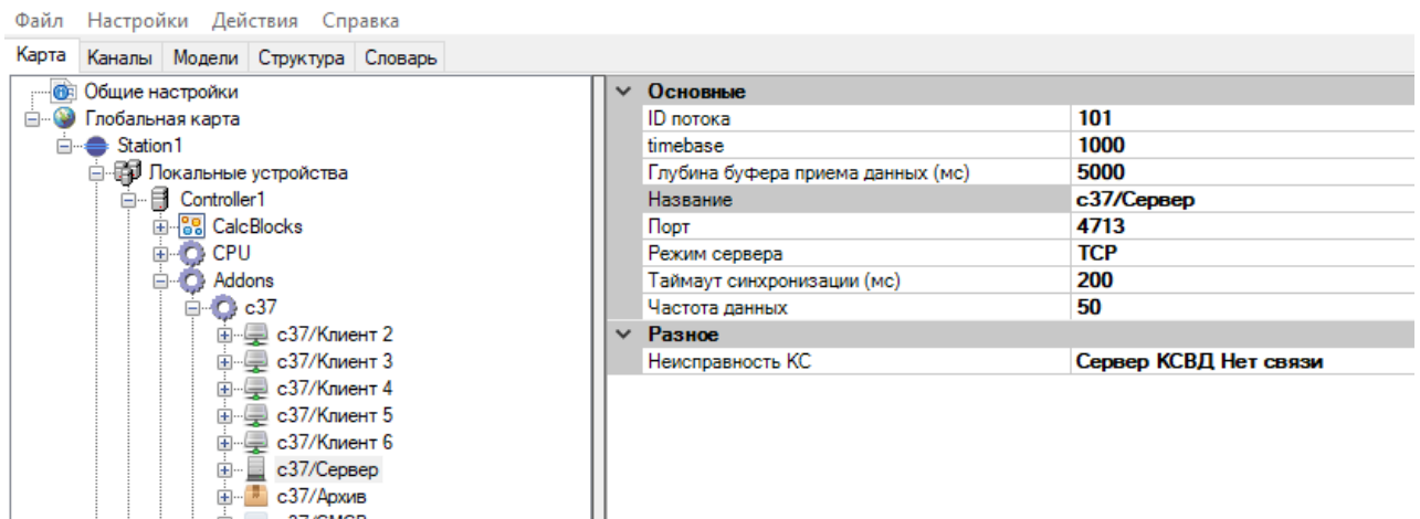
Рисунок 419. Настройка сервера С37.118
