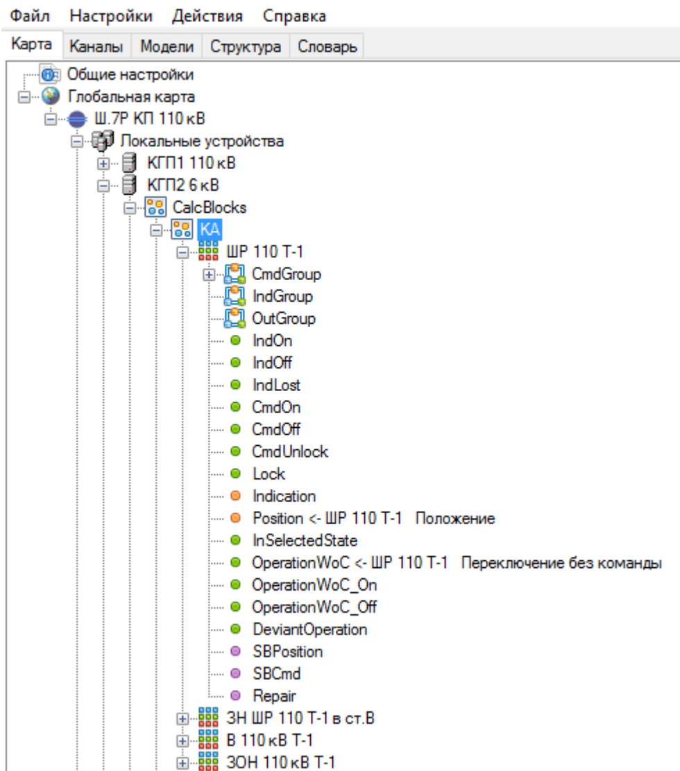
Рисунок 46б. Результат импорта группы КА
