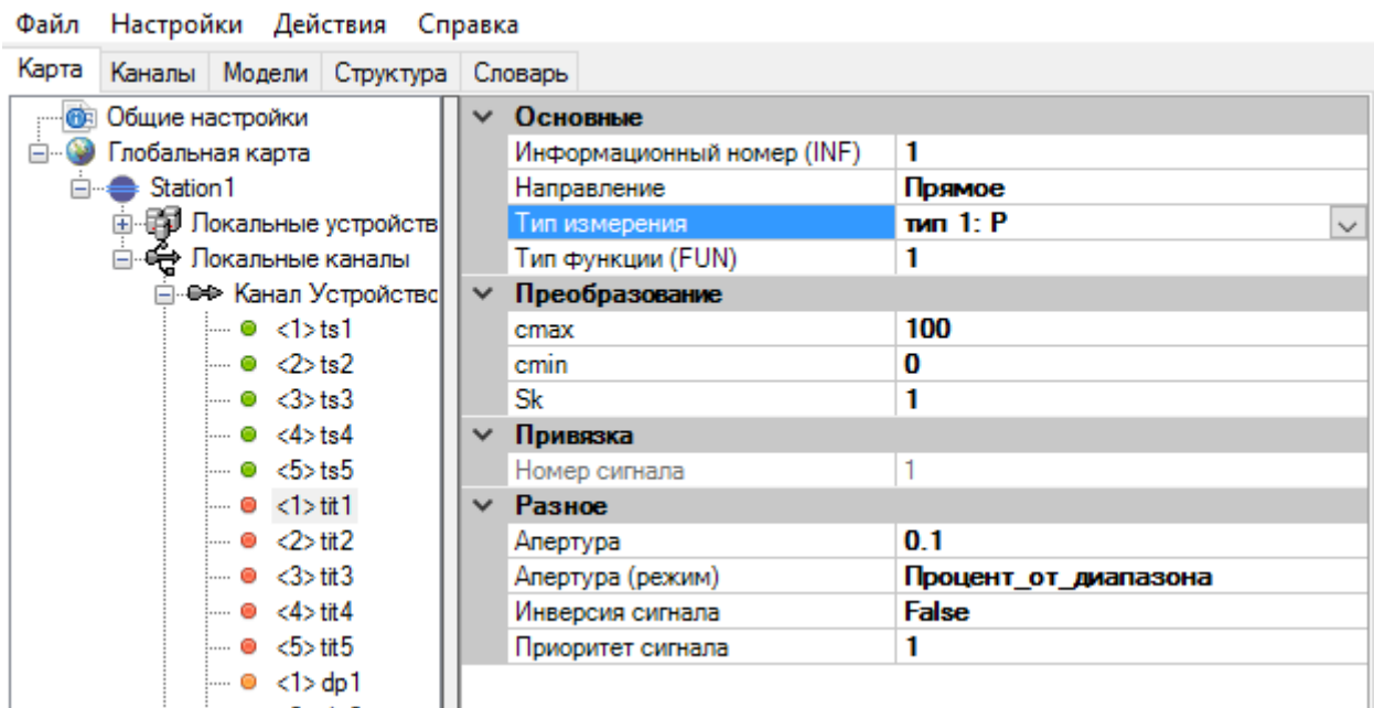
Рисунок 249. Настройки переменных канала связи МЭК60870-5-103
