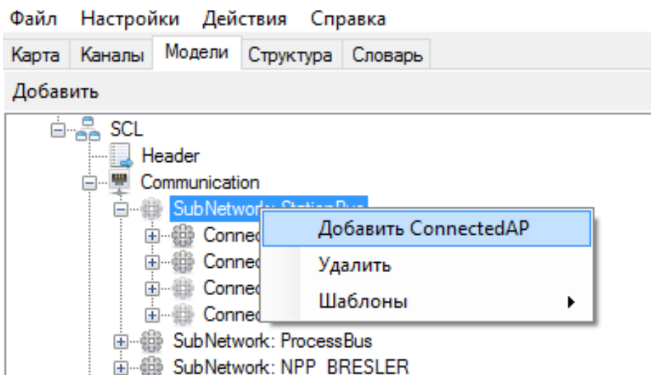
Рисунок 369. Объектная модель. Добавление ConnectedAP
