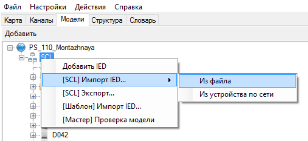
Рисунок 343. Объектная модель. Импорт IED-устройства
