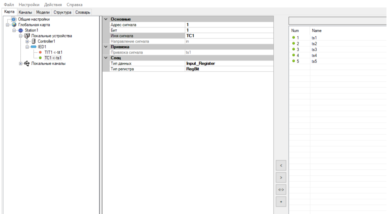
Рисунок 205. Привязка переменных к IED Modbus TCP
