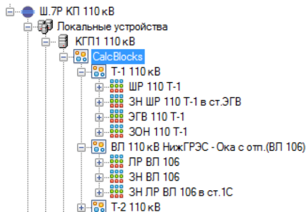
Рисунок 123. Группировка функциональных блоков
