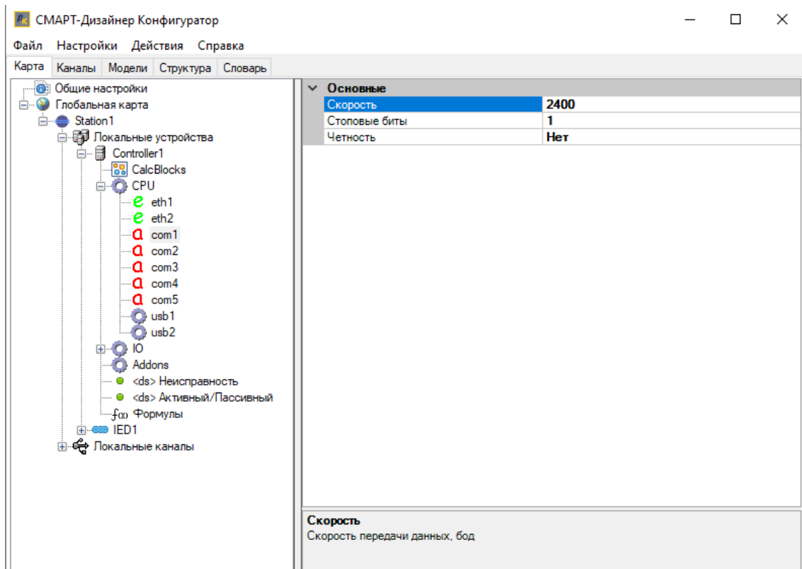
Рисунок 222. Настройка порта на контроллере для связи с ИБП
