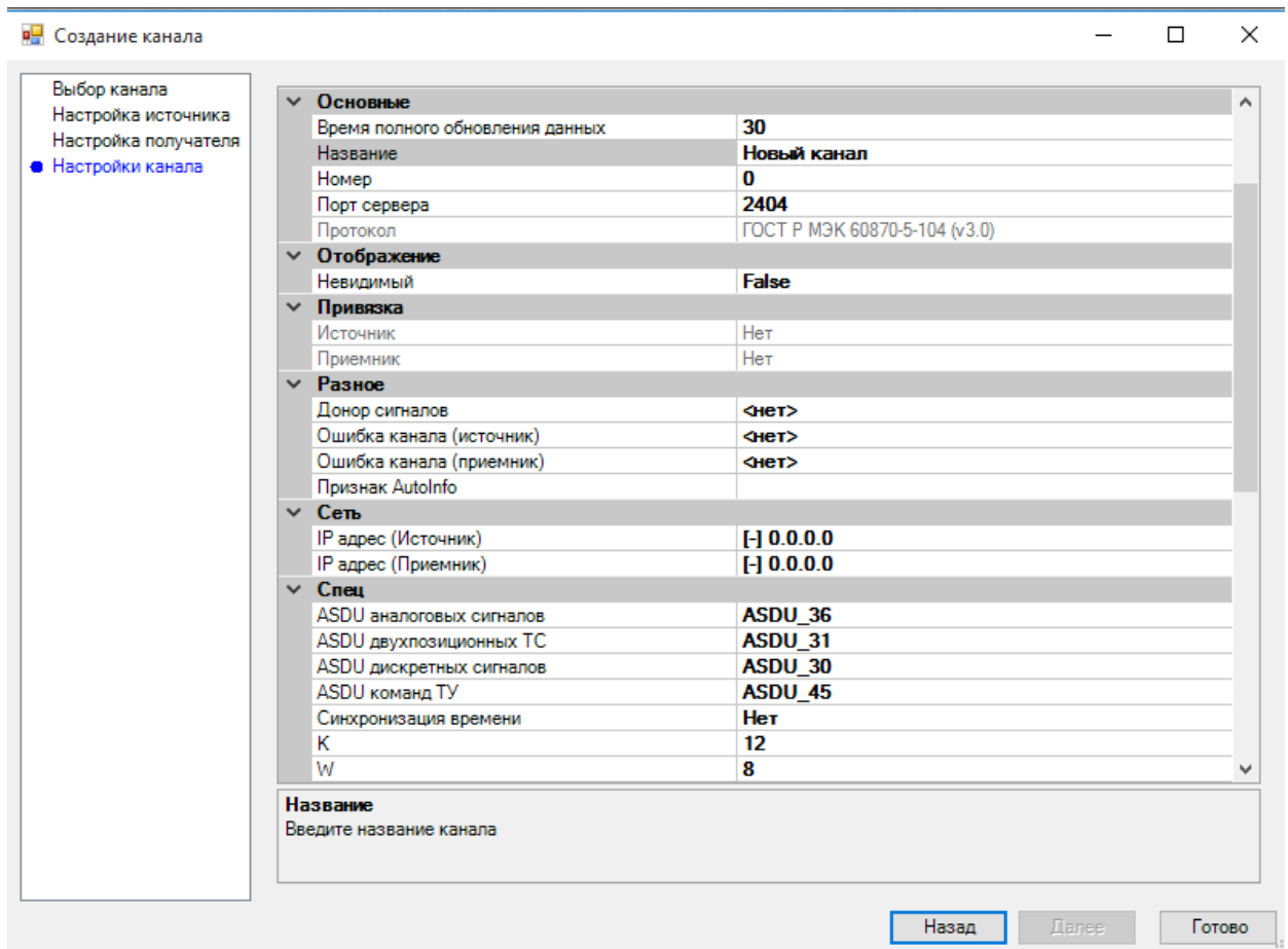
Рисунок 228. Конфигурирование настроек канала
