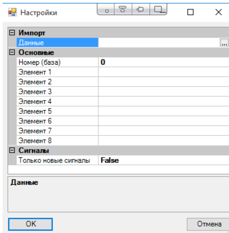
Рисунок 456. Импорт из шаблона
