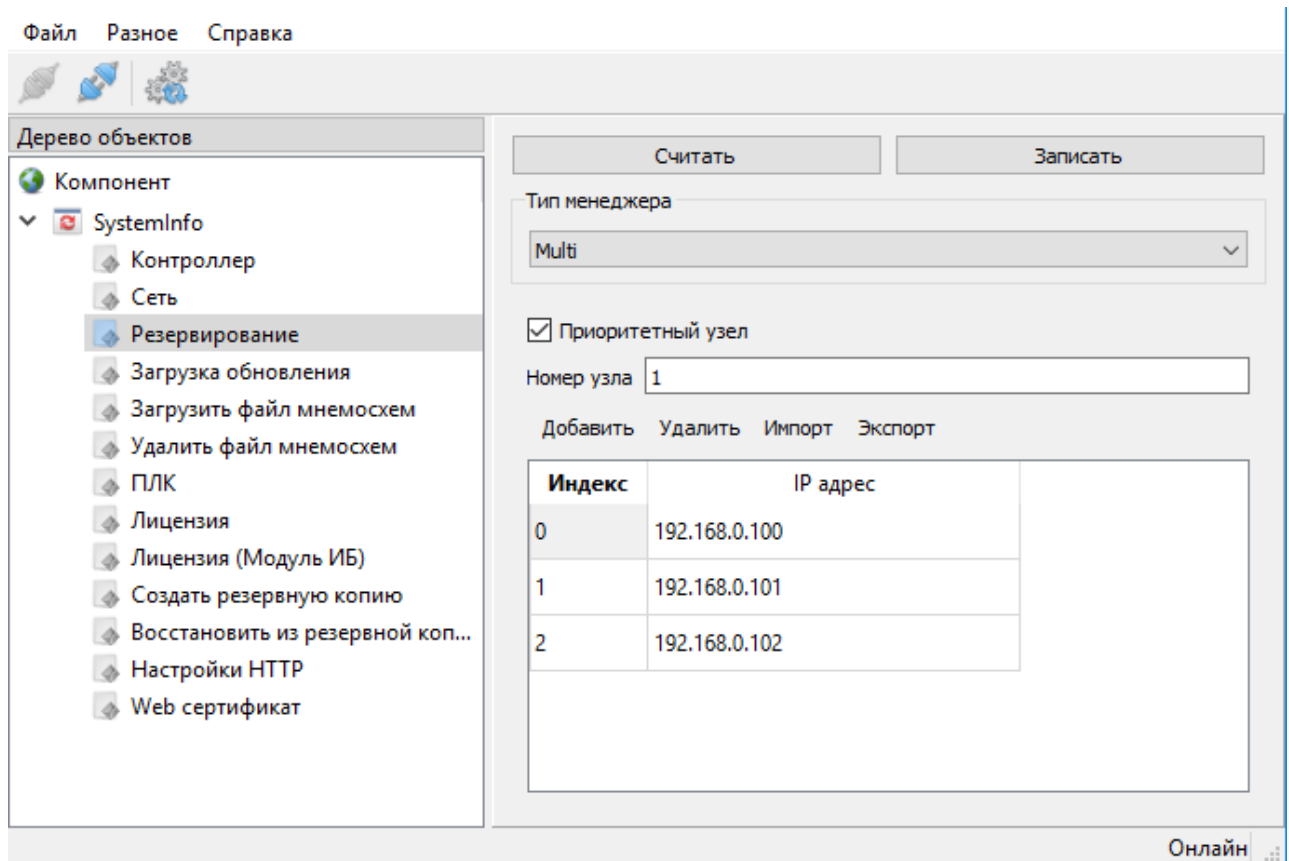
Рисунок 535. Настройки режима «Multi»
