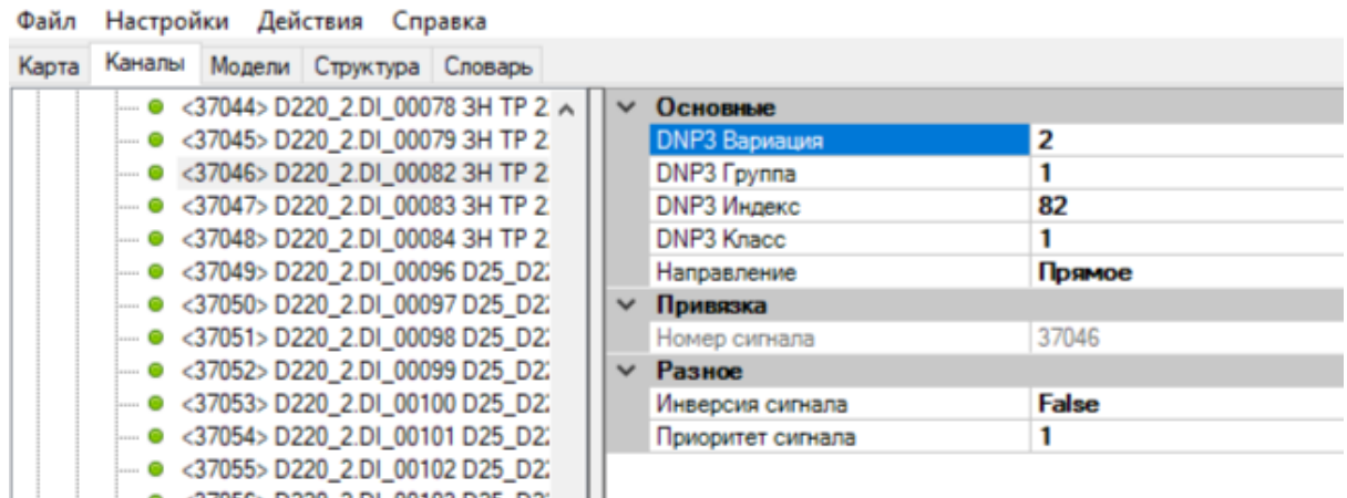
Рисунок 270. Настройки ТС канала связи DNP3
