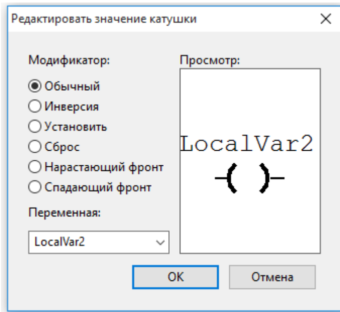
Рисунок 606. Смарт-Дизайнер ПЛК. Программа LD. Добавление катушки
