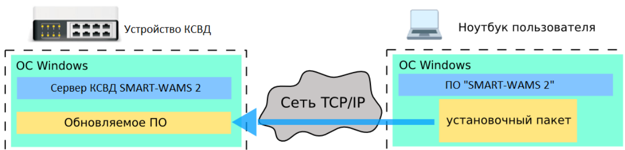
Рисунок 3 - Стенд для тестирования обновления программного обеспечения.
