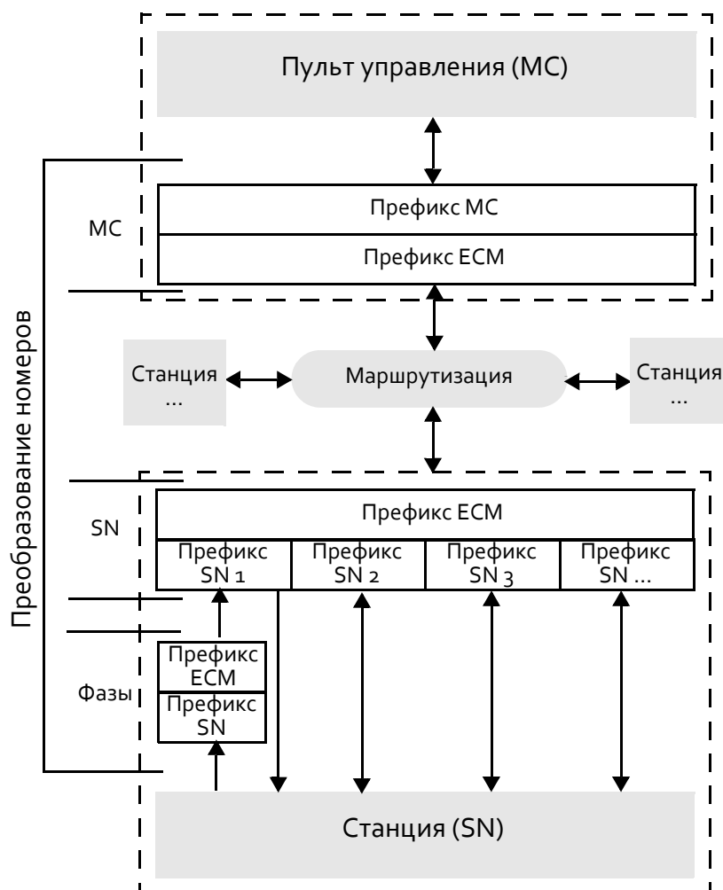
Рис. 3.1. Алгоритм преобразования номеров
