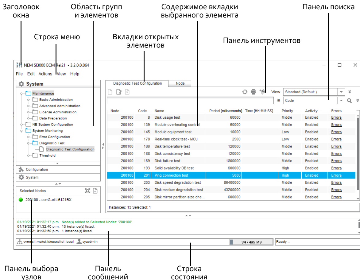
Рис. 2.2. Элементы главного окна менеджера NEM
