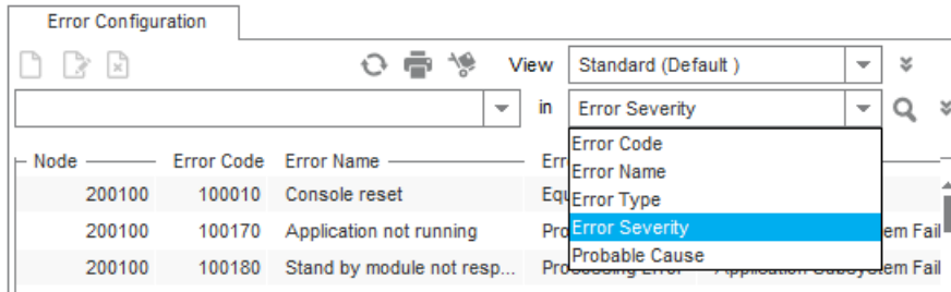
Рис. 2.15. Выбор параметра для простого поиска
