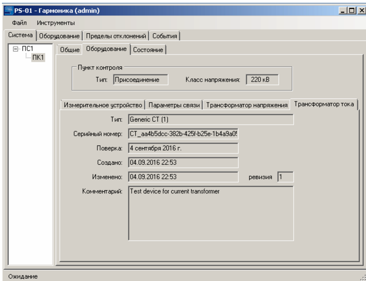
Рисунок 14. Трансформатор тока
