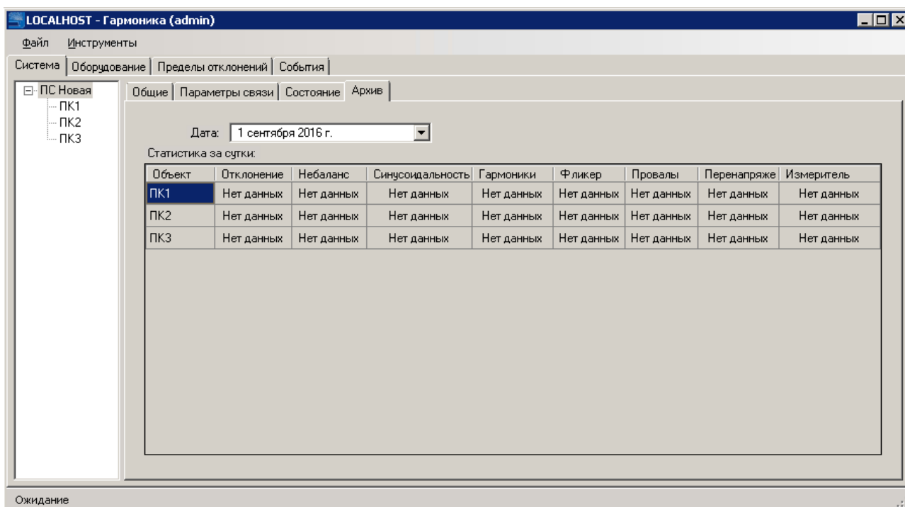
Рисунок 8. Закладка «Архив»
