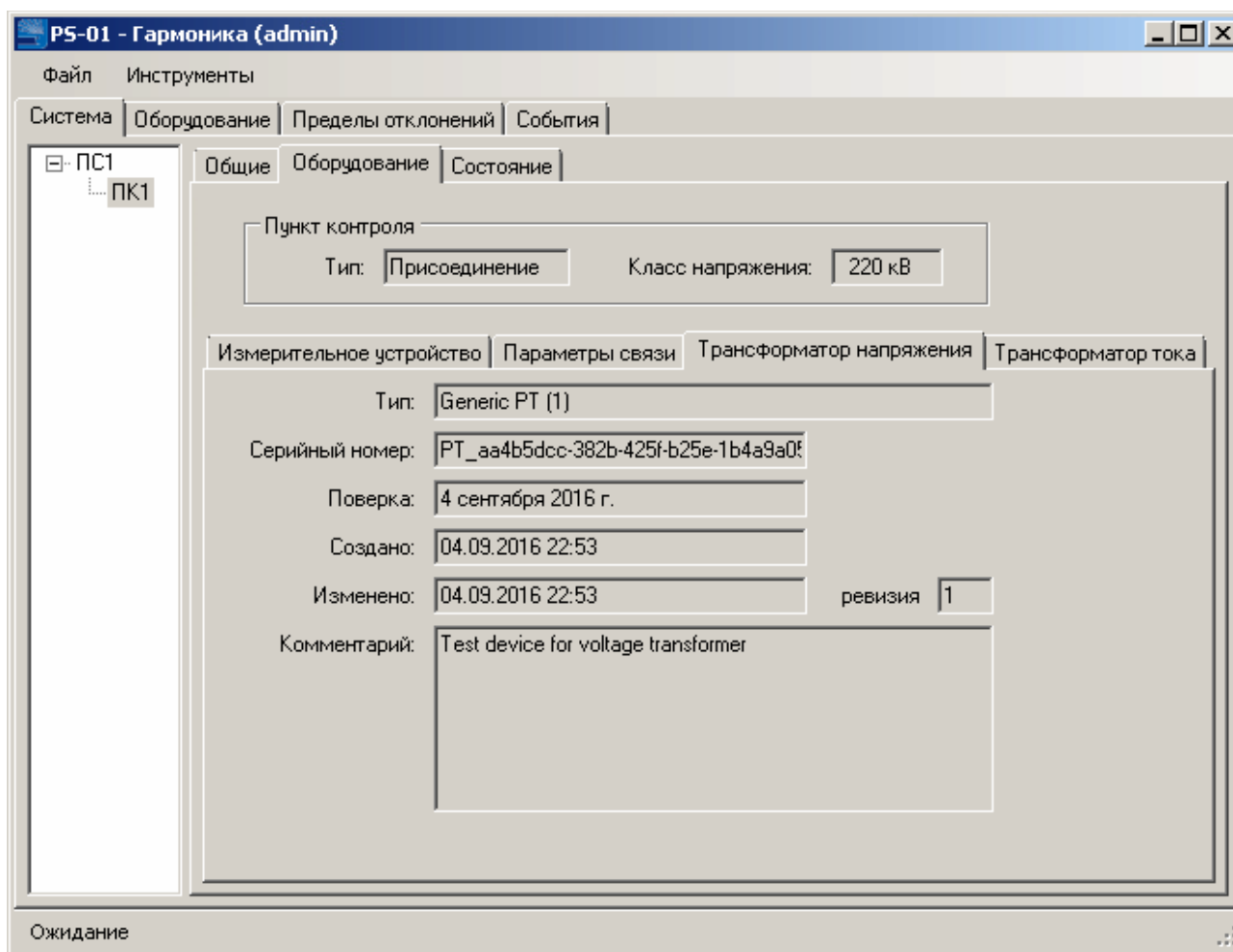
Рисунок 13. Трансформатор напряжения
