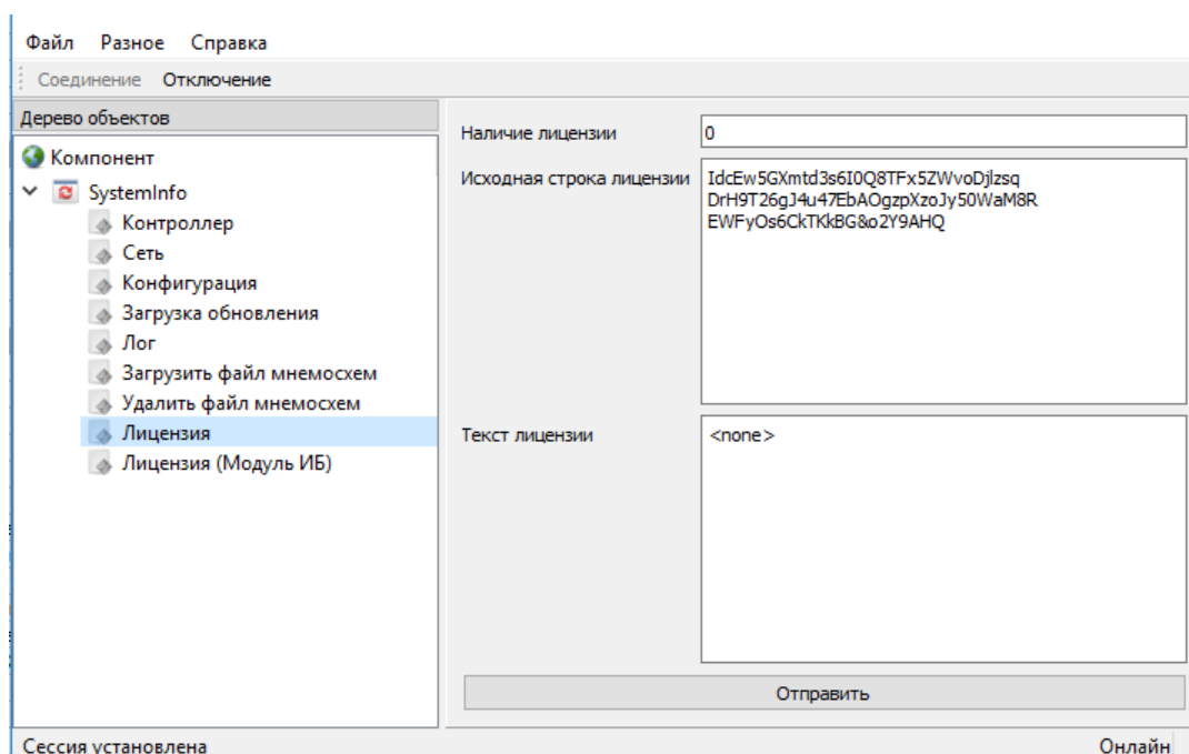
Рисунок 18. Установка лицензии
