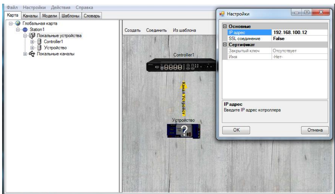
Рисунок 24. Загрузка конфигурации
