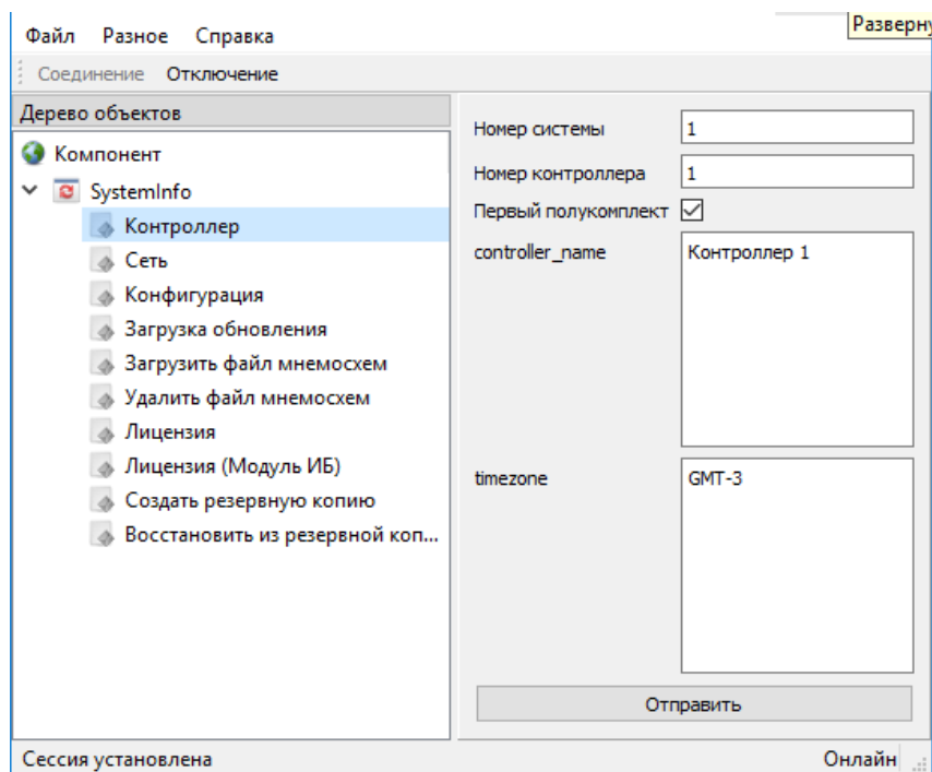
Рисунок 20. Установка идентификаторов контроллера
