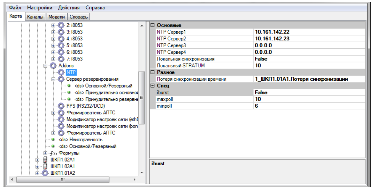
Рисунок 22. Настройка NTP
